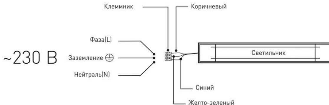
Рис.1. Схема подключения светильника к сети 230В.
