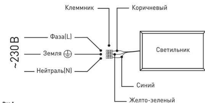
Рис.1. Схема подключения светильника SP0-7-50/ SP0-7-72 к сети 230В.
