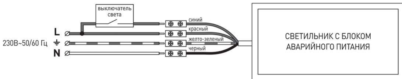
Рис.1. Схема подключения светильника
