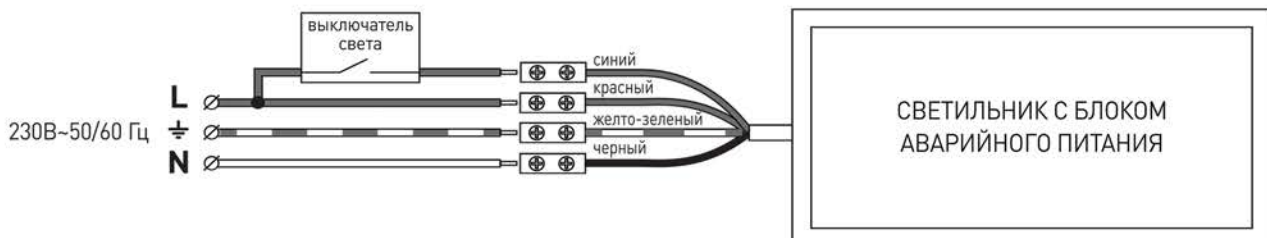
Рис.1. Схема подключения светильника к сети 230В.
