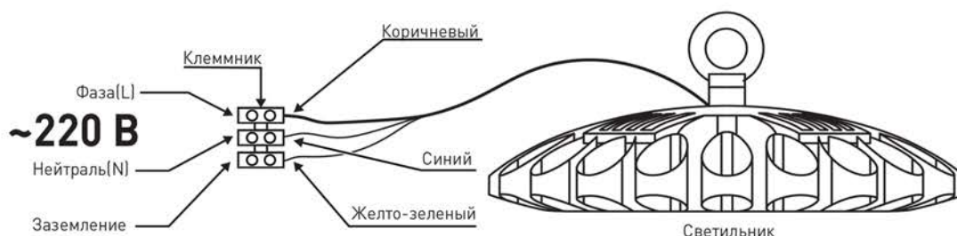
Рис.1. Схема подключения светильника к сети 220В.
