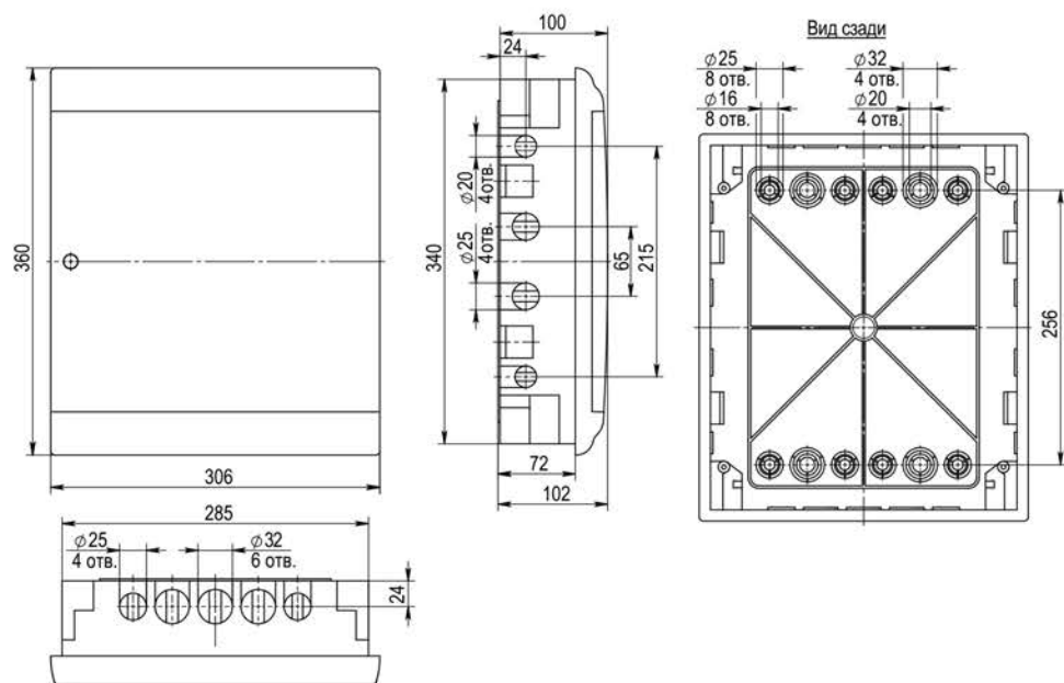
ЩРВ-П-24
