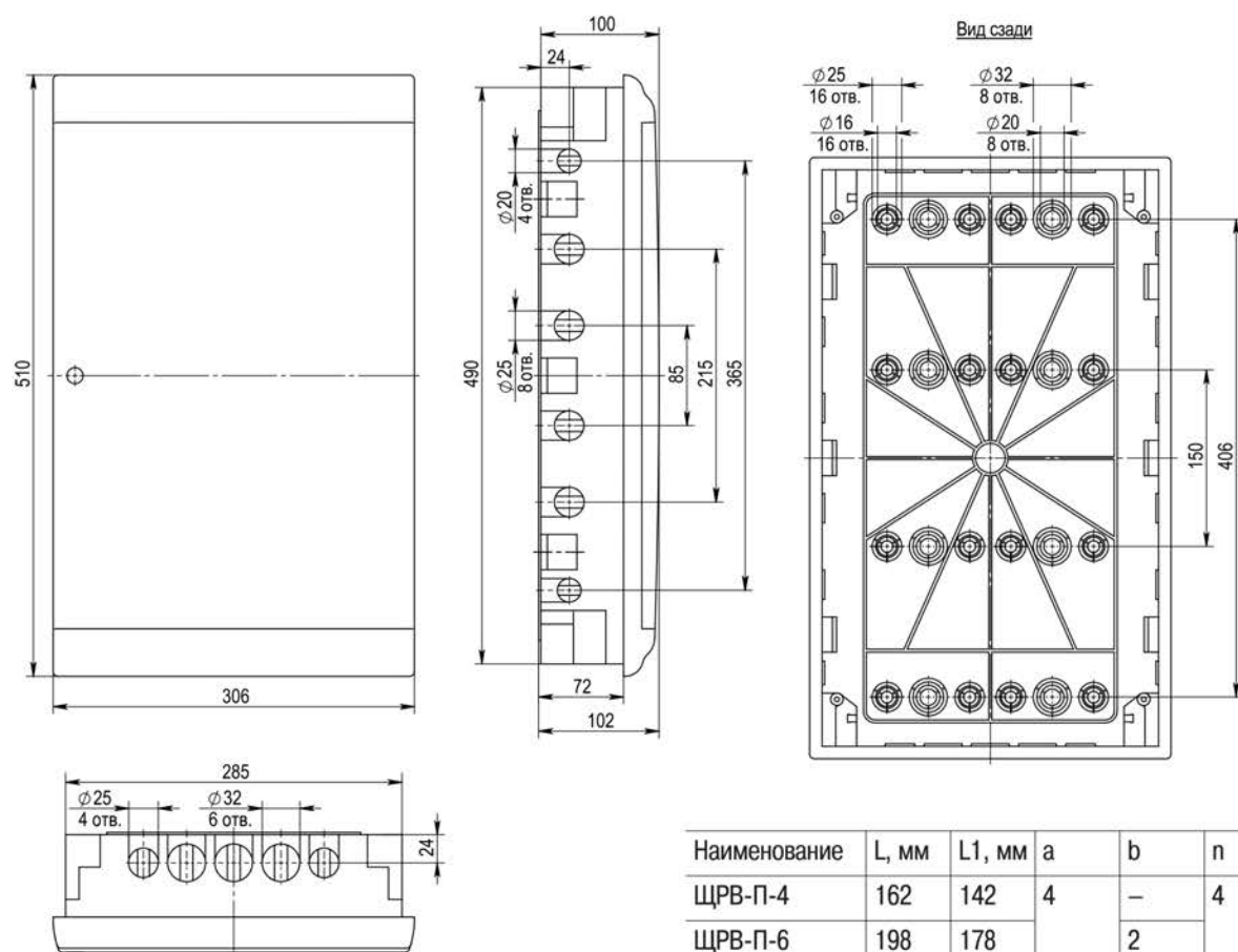
ЩРВ-П-36
