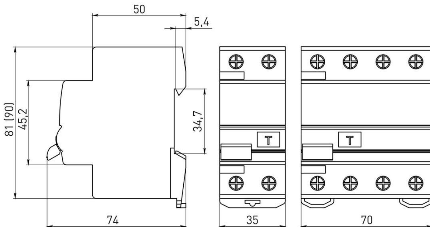
Рис. 1 - Габаритные размеры
