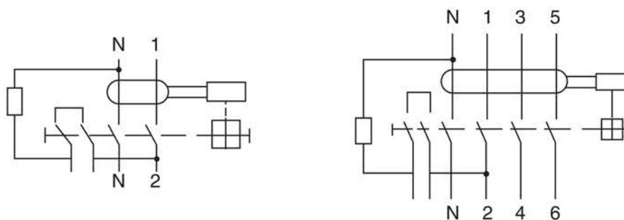
Рис. 2 - Схемы подключения
