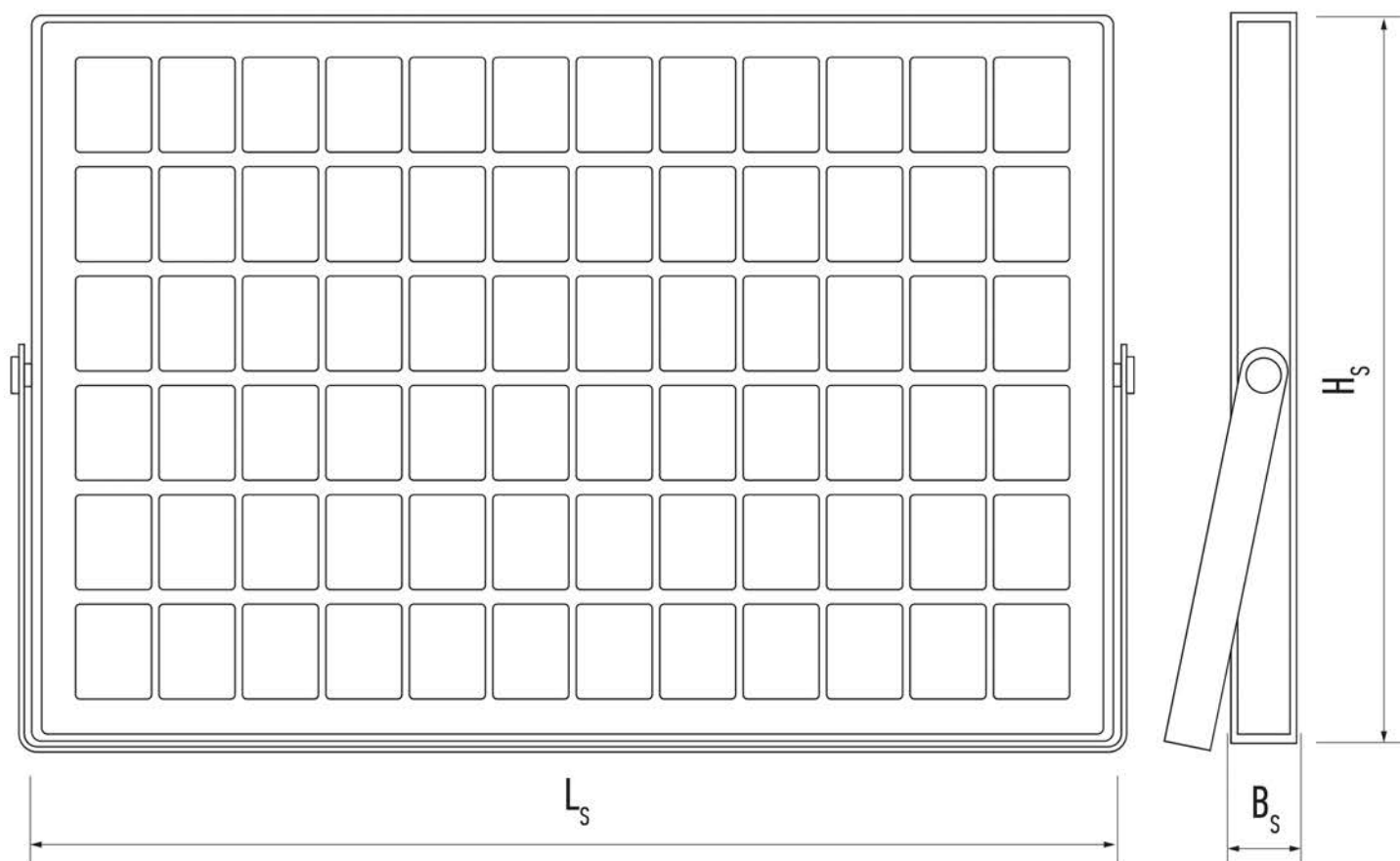
Рис. 3 Габаритные размеры солнечной панели
