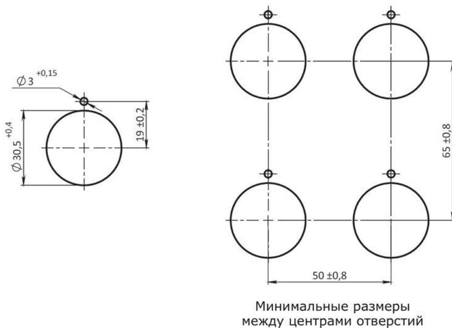
Рисунок 1 – Установочные размеры выключателей
