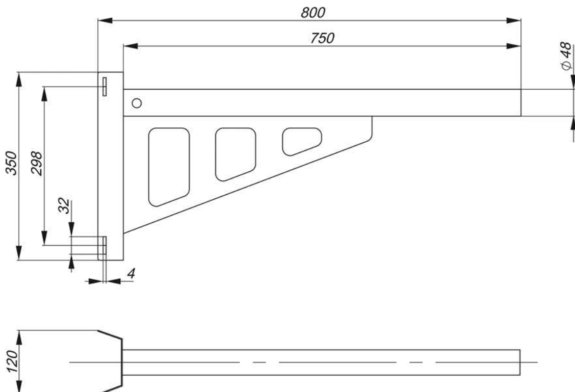
Рисунок 9 – Кронштейн LDKU0D-CR-48-0750-12-K03
