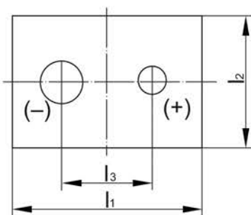
Рисунок 2 – Габаритные размеры 6LR61
