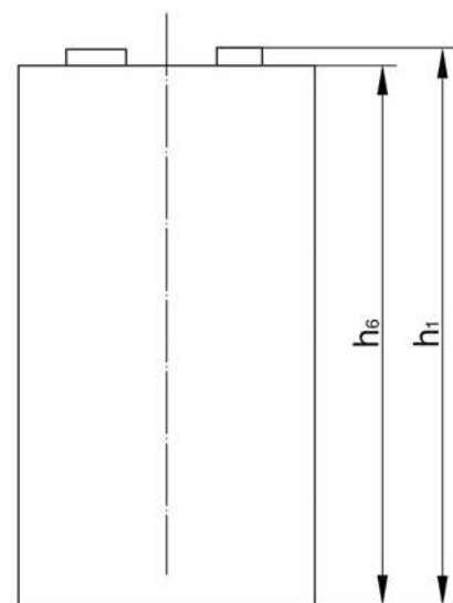
Рисунок 1 – Габаритные размеры LR03, LR6, LR14, LR20
