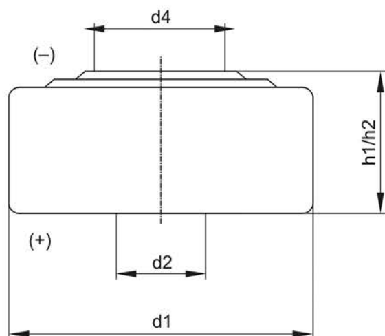
Рисунок 3 – Габаритные размеры LR44
