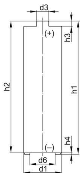
Рисунок 1 – Габаритные размеры LR03, LR6, LR14, LR20
