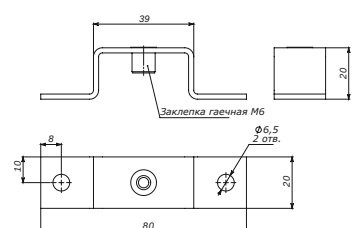
Кронштейн 20 мм
