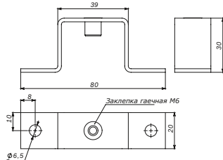
Кронштейн 30 мм
