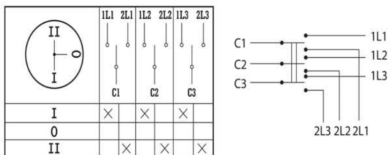
Рис. 16 - Пакетный переключатель 3-полюсный на 2 направления
