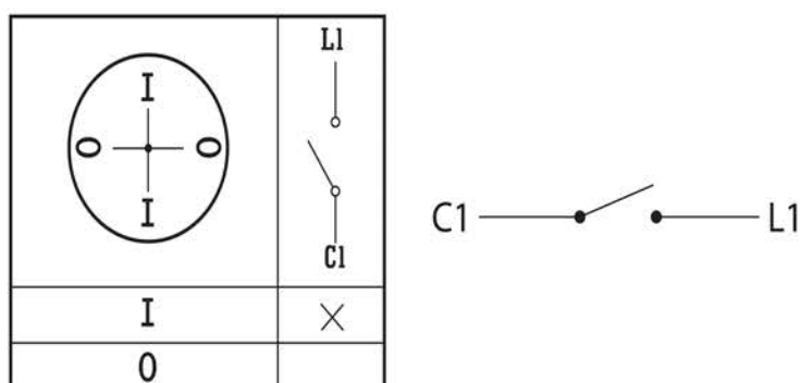
Рис. 10 - Пакетный выключатель 1-полюсный
