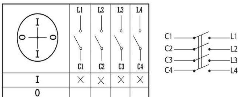
Рис. 13 - Пакетный выключатель 4-полюсный
