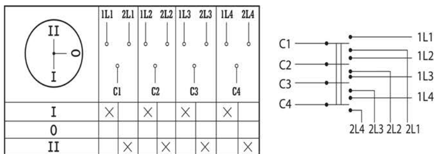
Рис. 17 - Пакетный переключатель 4-полюсный на 2 направления
