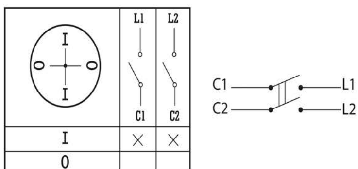
Рис. 11 - Пакетный выключатель 2-полюсный
