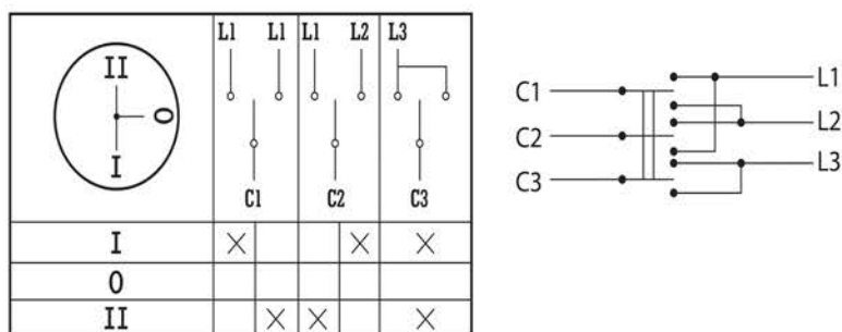
Рис. 18 - Пакетный переключатель 3-полюсный реверсный
