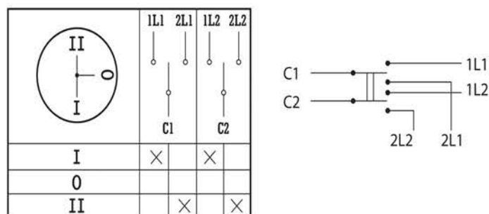
Рис. 15 - Пакетный переключатель 2-полюсный на 2 направления
