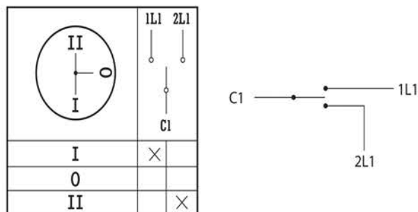
Рис. 14 - Пакетный переключатель 1-полюсный на 2 направления
