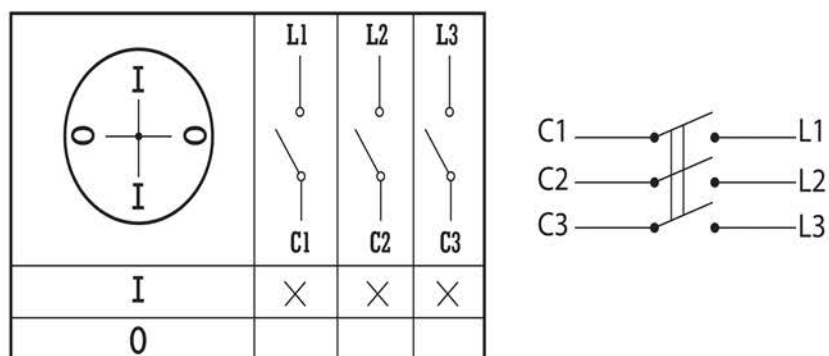
Рис. 12 - Пакетный выключатель 3-полюсный
