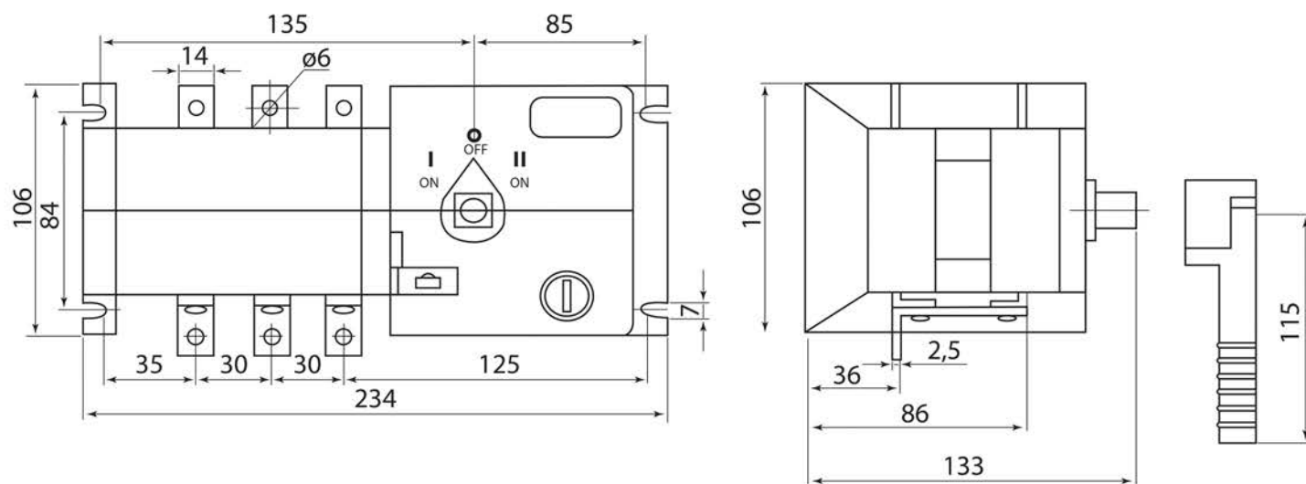
Рисунок 1. Габаритные размеры АВР-ПНУ, мм
