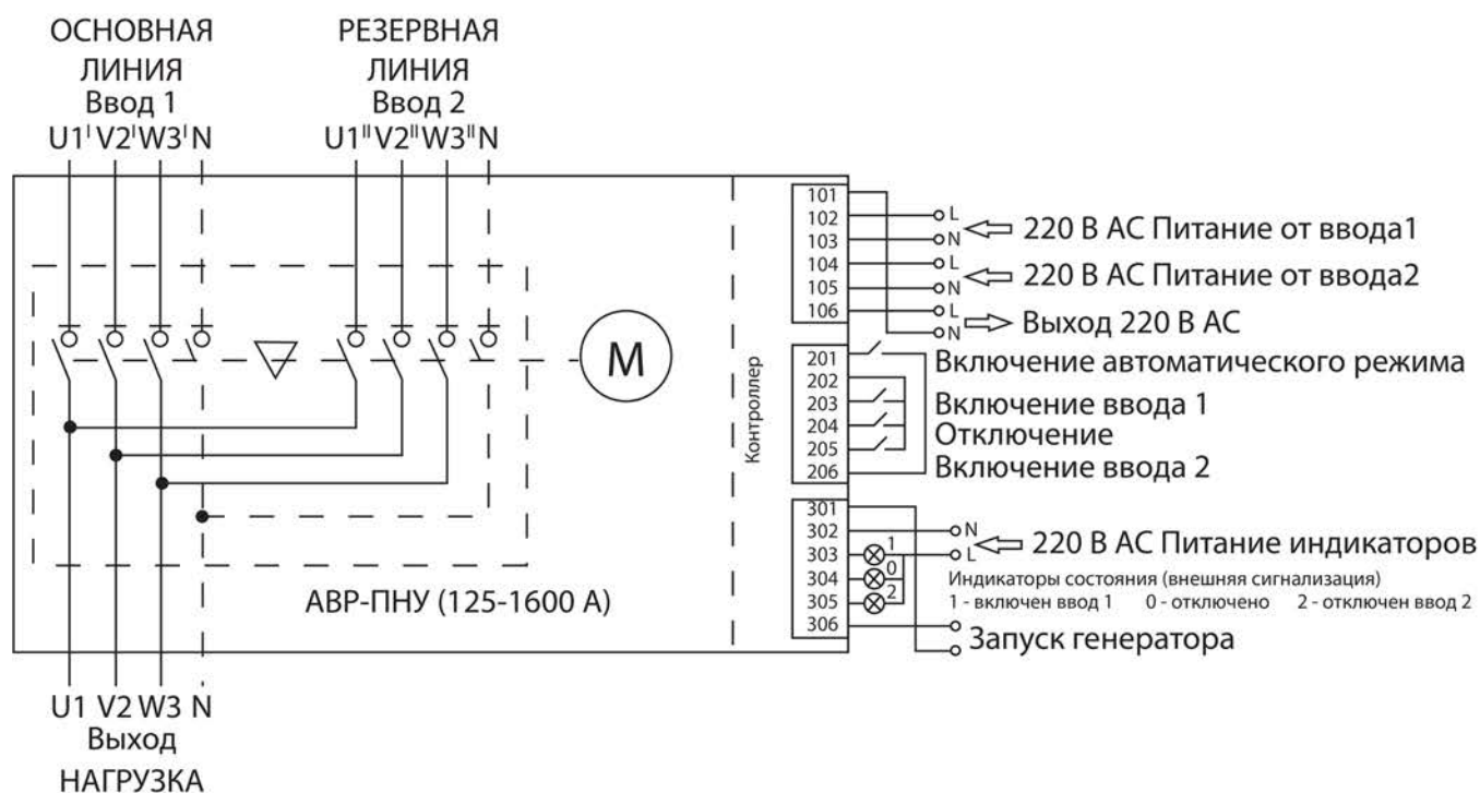
Рисунок 3. Схема подключения АВР-ПНУ 32-1600 А
