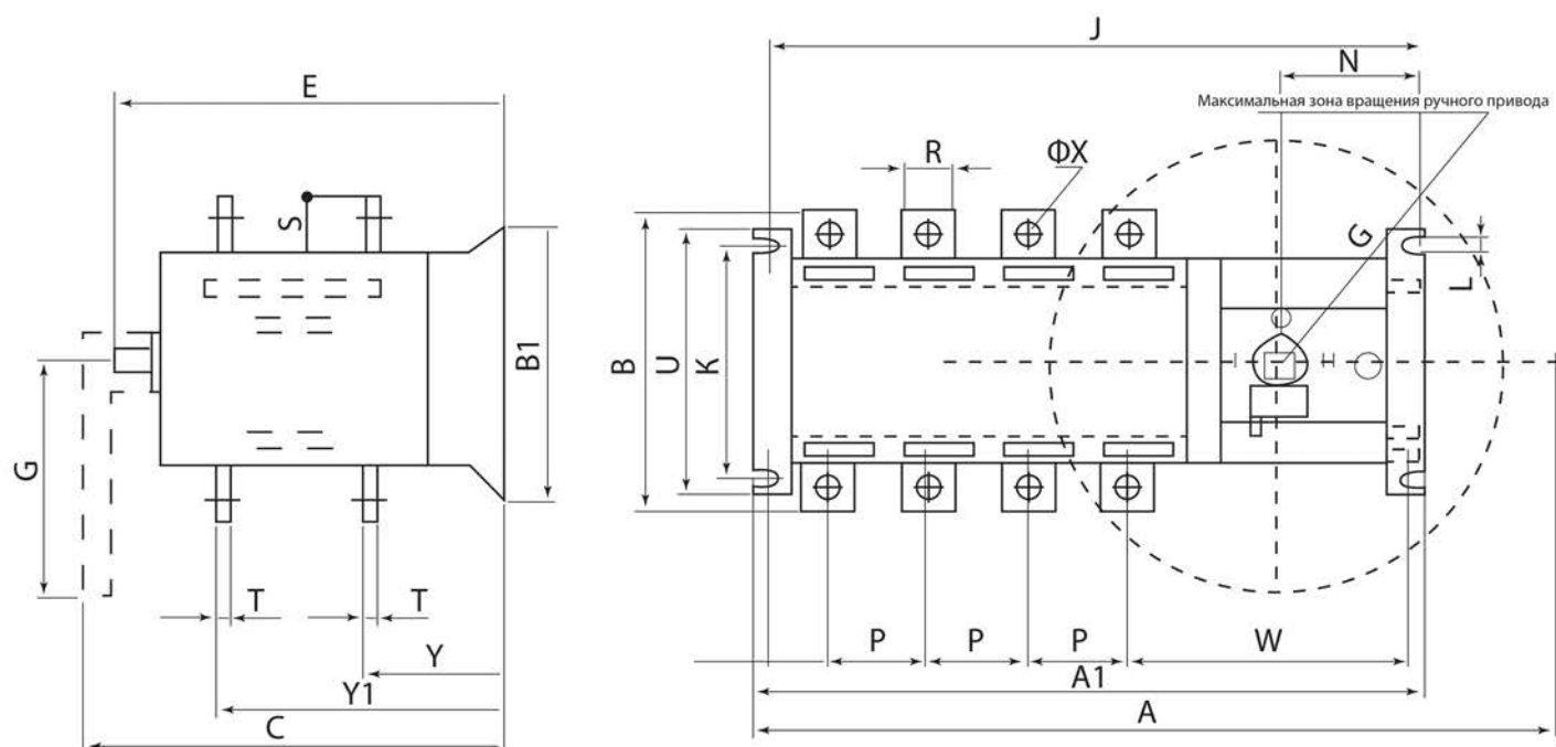
Рисунок 2. Габаритные размеры АВР-ПНУ 125-1600 А, мм
