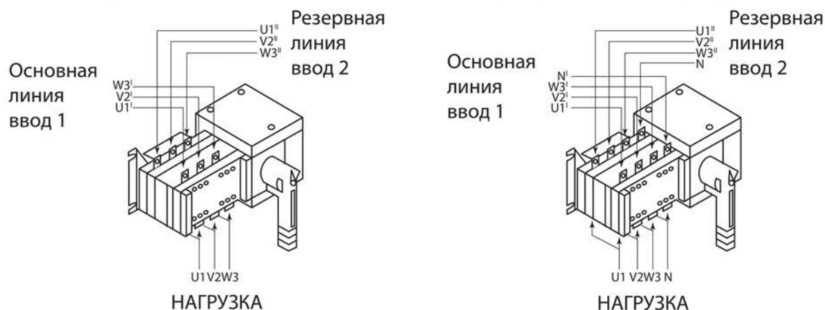
Рисунок 5. Подключение силовых цепей АВР-ПНУ
