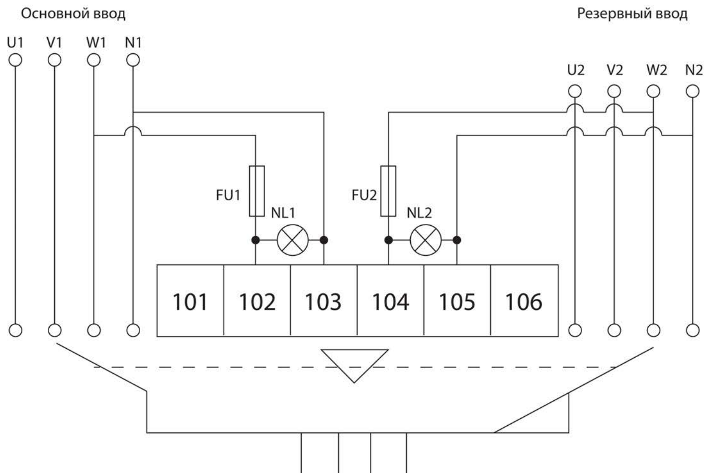
Рисунок 6. Подключение питания цепей управления АВР-ПНУ
