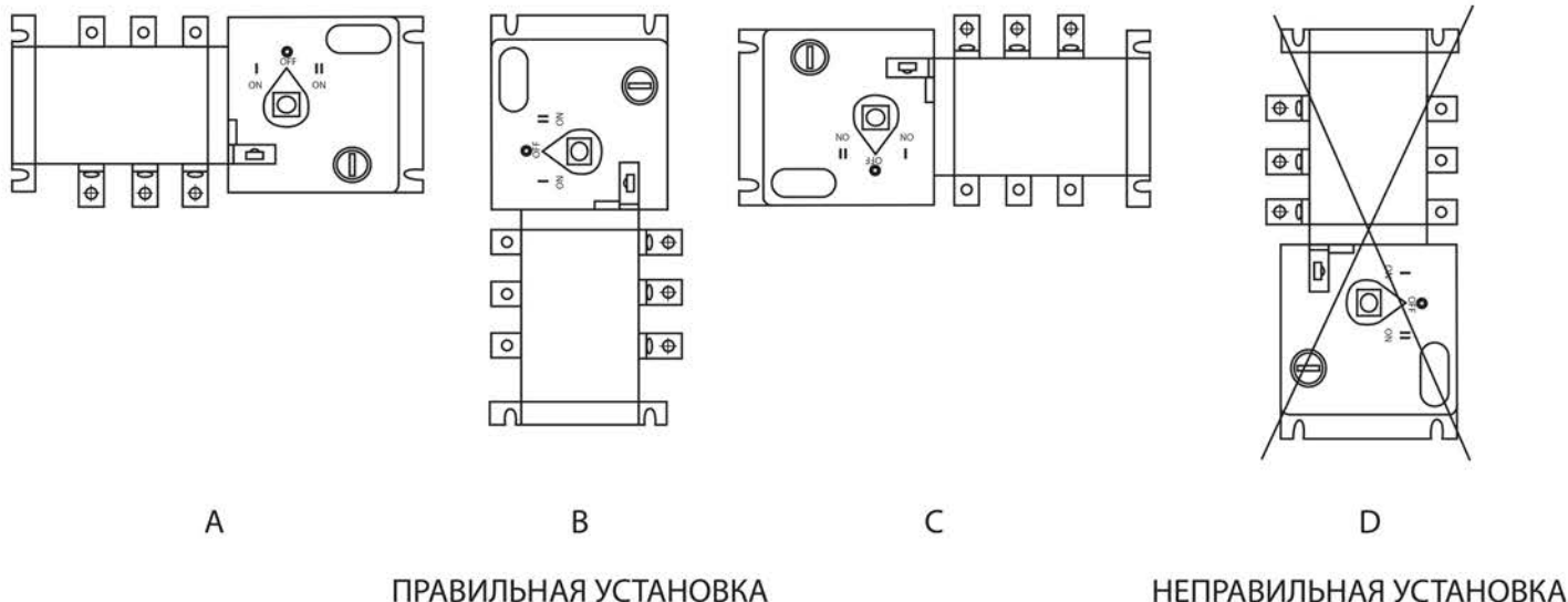
Рисунок 4. Варианты установки устройства АВР-ПНД
