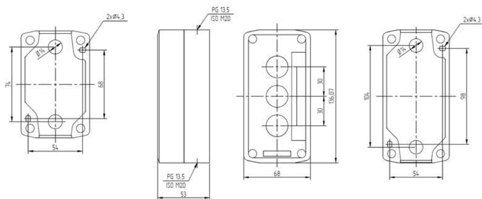
Масса – 0,238 кг Рисунок А.4 – Посты OptiSignal D22 A5-BD-3
