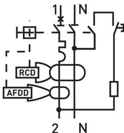
Рис. 4 – Типовая схема подключения
