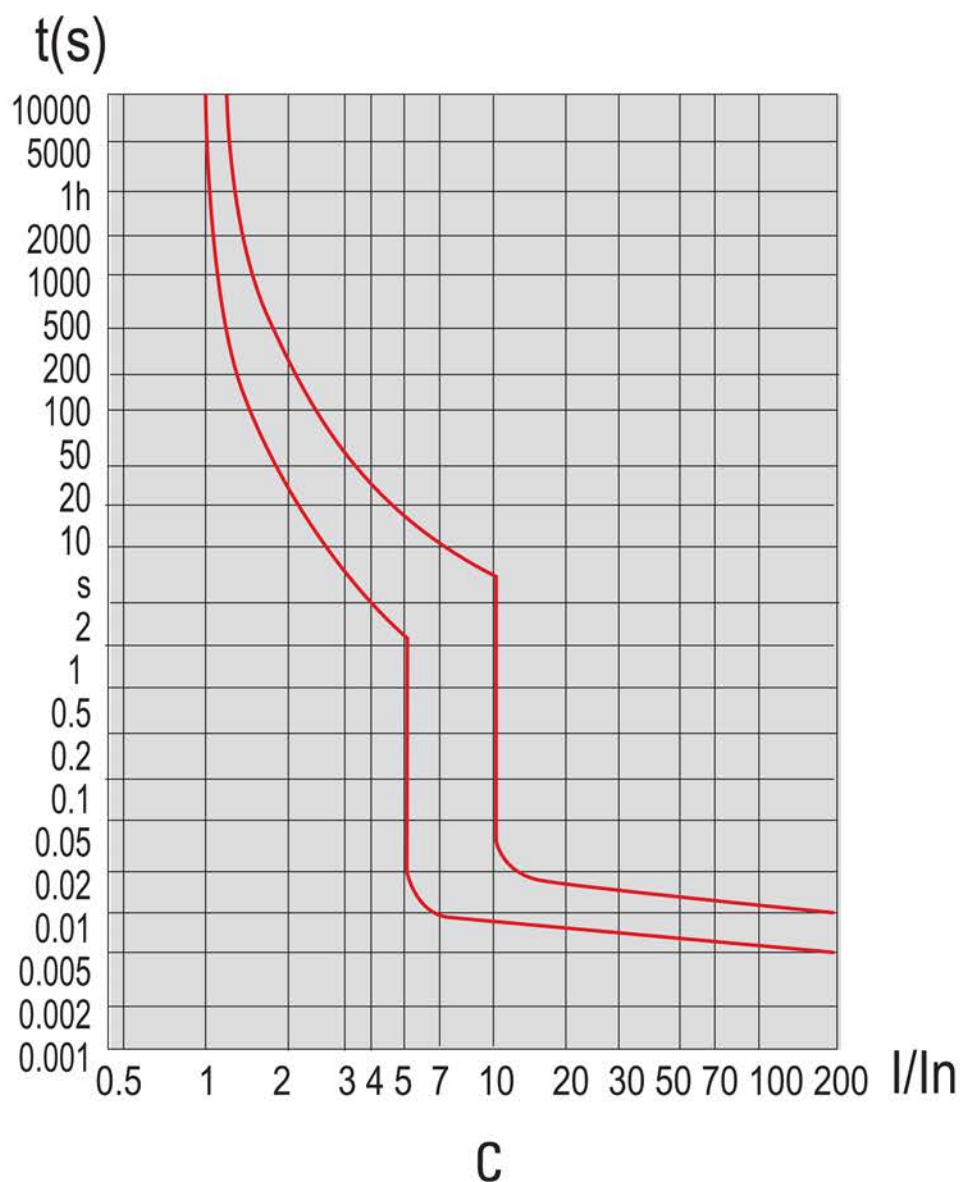
Рис. 2 – Время-токовые характеристики
