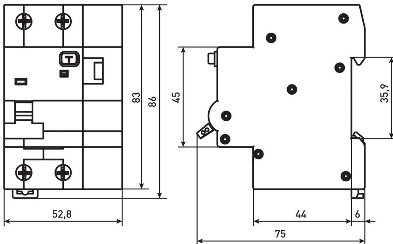
Рис. 3 – Габаритные размеры
