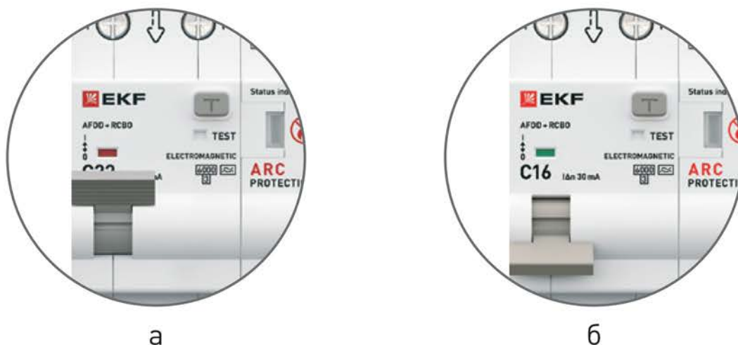
Рис. 5 – Механический указатель физического положения контактов
