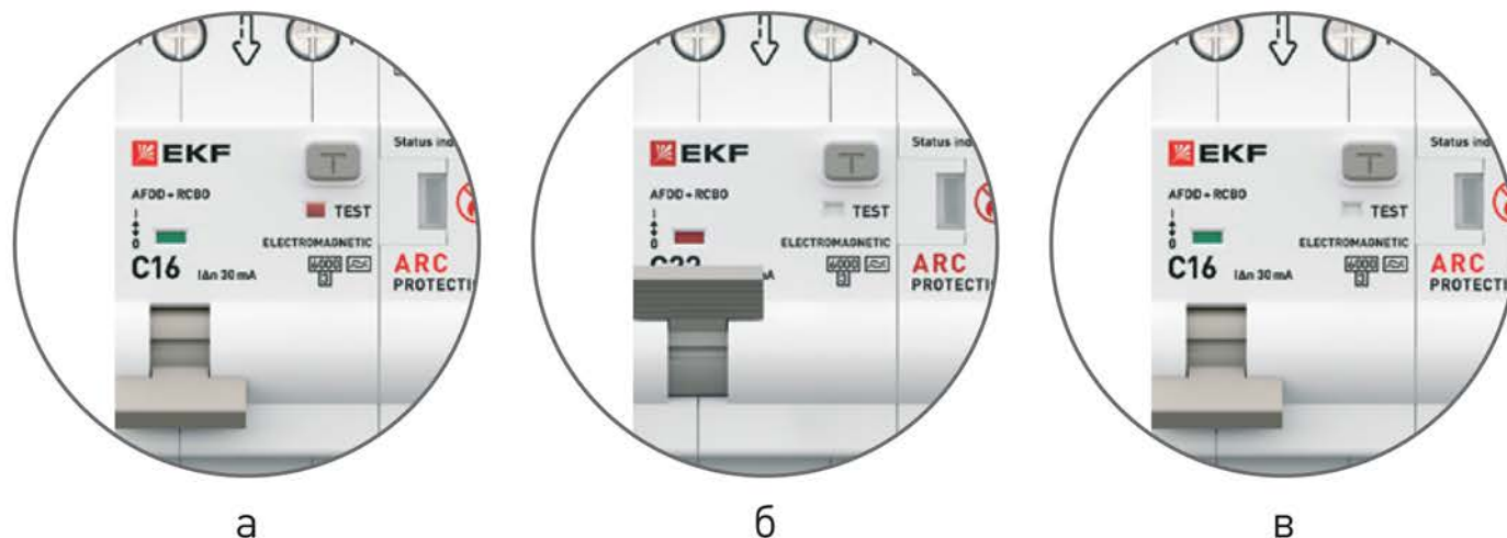
Рис. 6 – Механический указатель срабатывания от токов утечки
