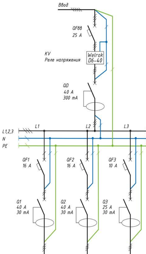
Схема 3. Вариант электрической схемы с тремя однофазными нагрузками
