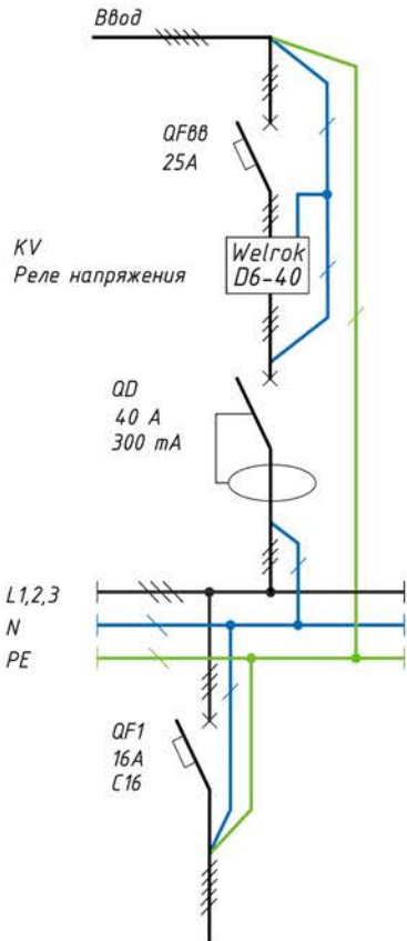
Схема 2. Вариант электрической схемы с трехфазной нагрузкой
