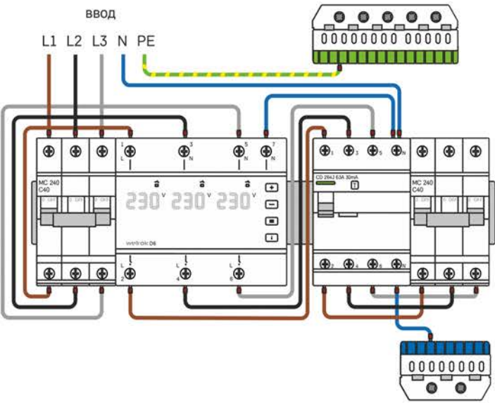
Схема 1. Монтажная схема
