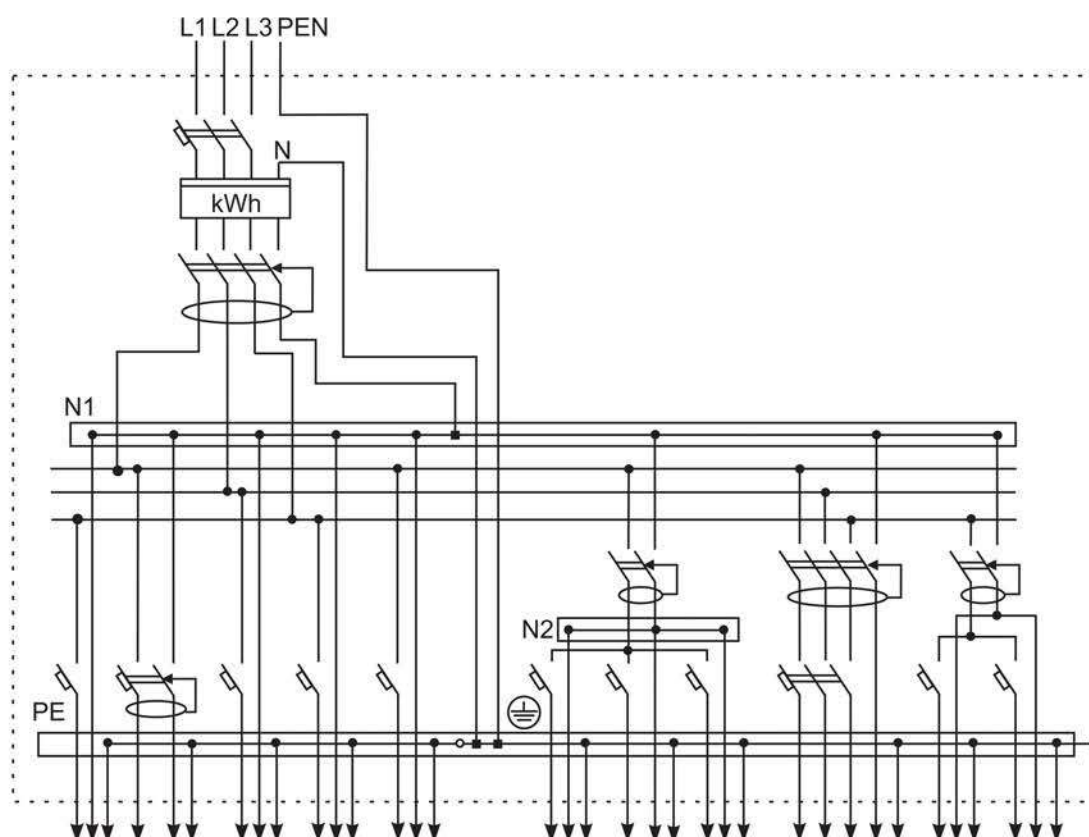
Рисунок 7. Схема квартирного учетно-группового щитка (для коттеджа)
