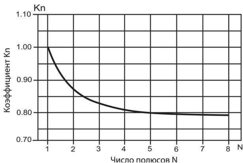
Рисунок 3. График зависимости коэффициента K_n от числа полюсов
