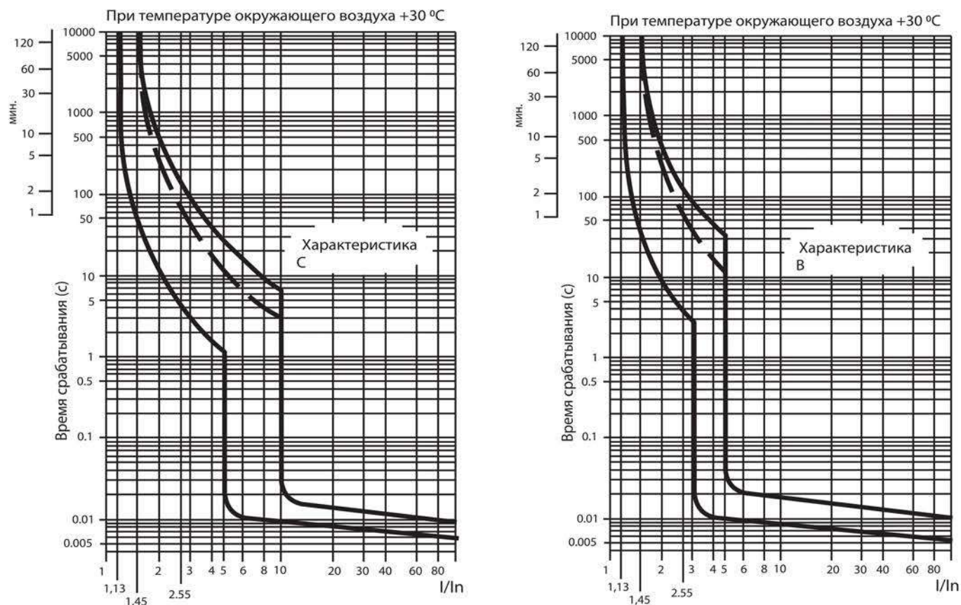
Рисунок 2. Время-токовые характеристики выключателей
