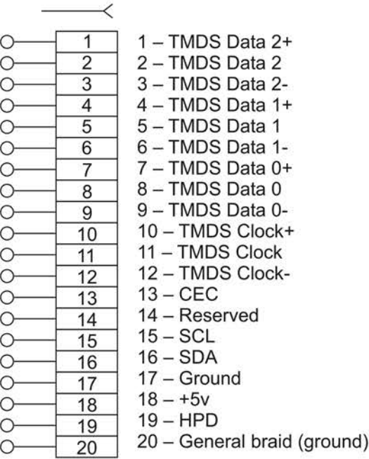
e) розетка / socket / priză HDMI
