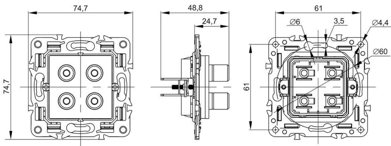
ф) аудио розетка / audio socket / акустикалы розетка / priza de acustică
