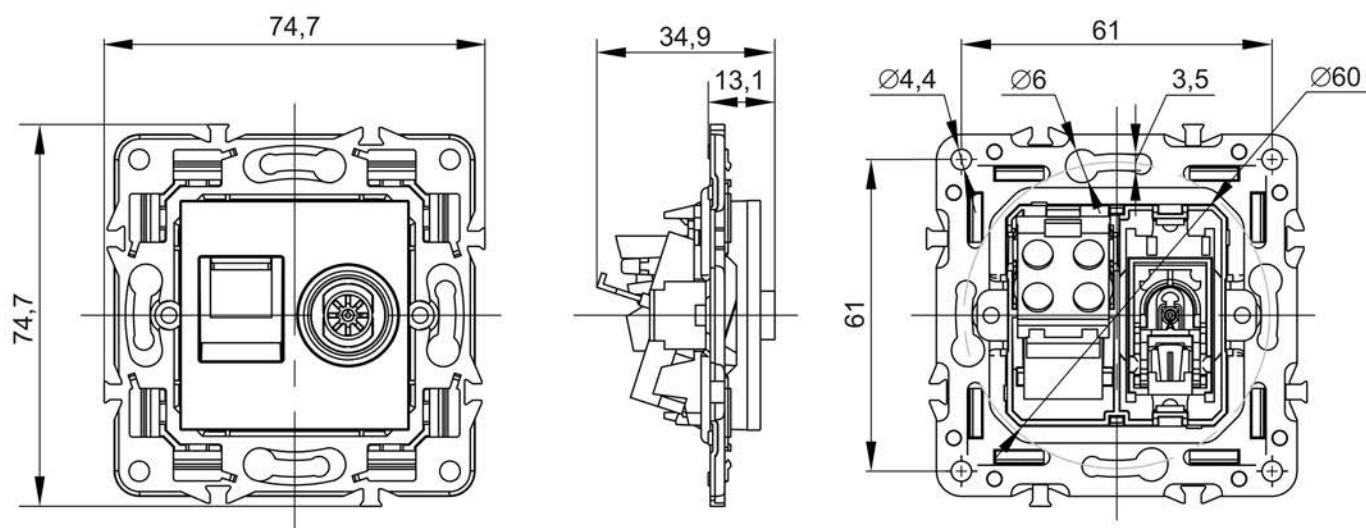
е) двойные розетки / double sockets / қос розеткалары / prize duble (RJ45+TV)
