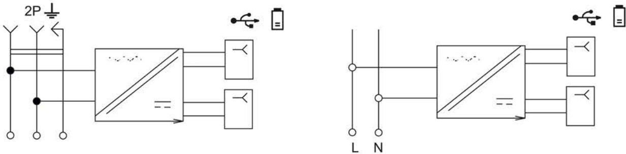
е) Розетка сетевая с розеткой USB type C / Power socket with USB type C socket / USB Type C розеткасы бар желілік розетка / Priză de rețea cu priză USB tip C ф) розетка / socket / prizele USB type A + type A / USB type A + type C
