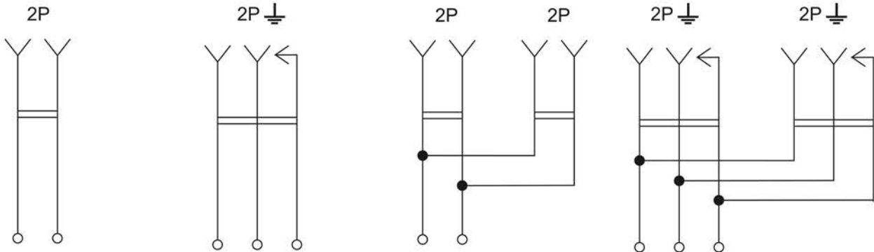
а) одноместная / single / жалғыз / singur б) одноместная с заземлением / single with grounding / жерге қосылатын жалғыз / single cu împământare в) двухместная / double / қосарлы / dublu г) двухместная с заземлением / double with grounding / жерге қосу арқылы қос / dublu cu împământare
