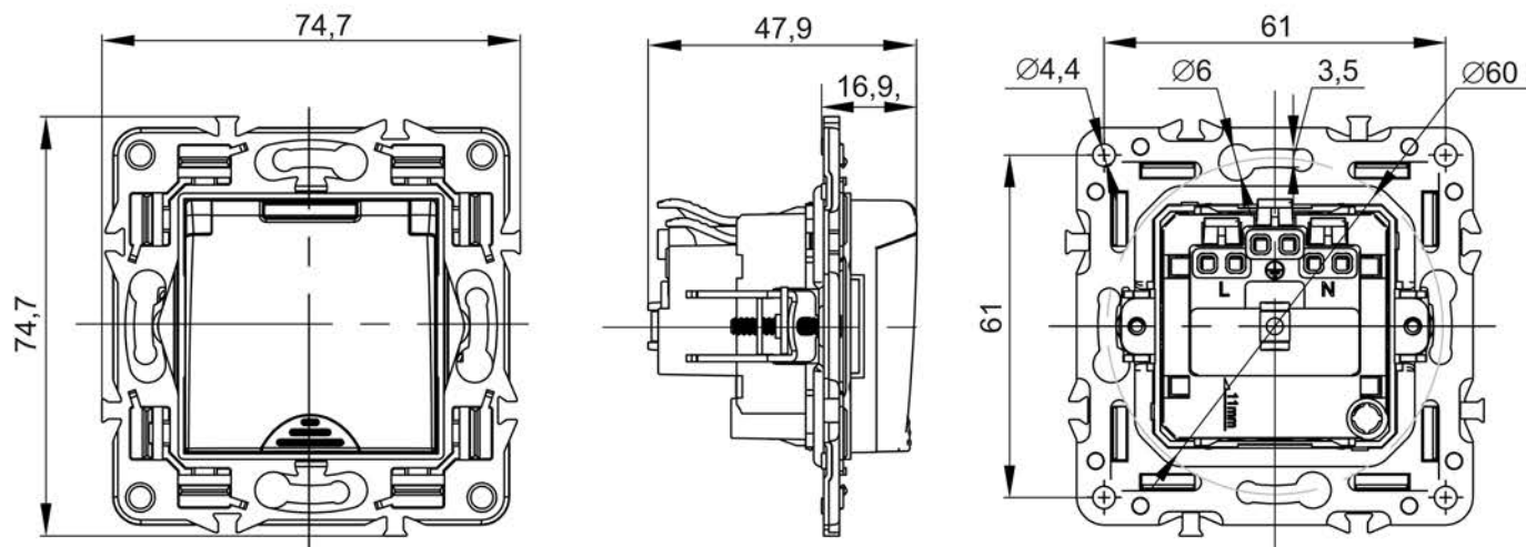
c) сетевые розетки с крышкой IP44 / sockets with cover IP44 / IP44 қақпағы бар желілік розеткалар / prize de retea cu capac IP44
