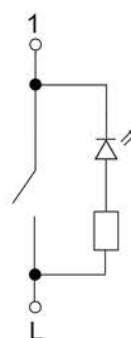
г) выключатель одноклавиш- ный с индикацией / 1-gang switch with indication / индикациясы бар бір пернелі ажыратқыш / intrerupator singură cu indicatie
