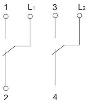
е) выключатель двухклавишный проходной / pass-through 2-gang switch / екі пернелі өтпелі ажыратқыш / intrerupator dublu de trecere prin
