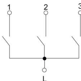
с) выключатель трехкла- вишный / 3-gang switch / үш пернелі ажыратқыш / comutator cu trei bande
