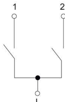
б) выключатель двухкла- вишный / 2-gang switch / екі пернелі ажыратқыш / intrerupator dublu
