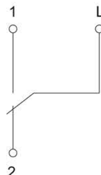
д) выключатель одноклавиш- ный проходной / pass-through 1-gang switch / бір пернелі өтпелі ажыратқыш / intrerupator singură de trecere prin
