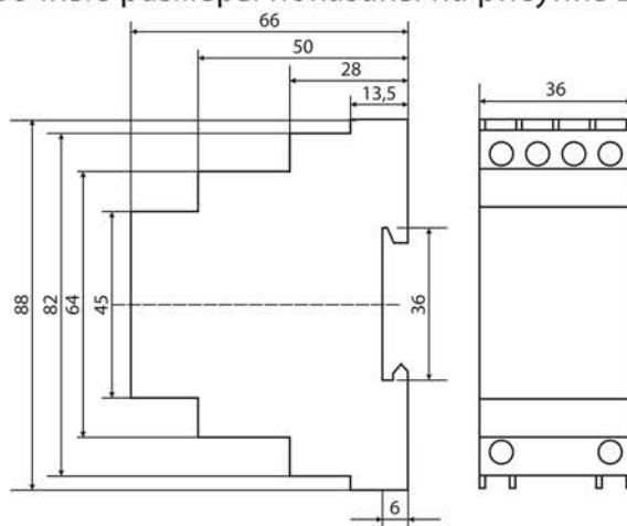
Рисунок 2. Габаритные и установочные размеры трансформаторов, мм
