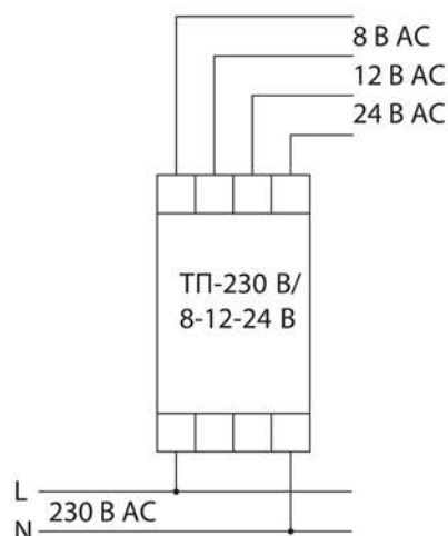
Рисунок 3. Схема подключения трансформатора ТП-230В/8-12-24В к сети
