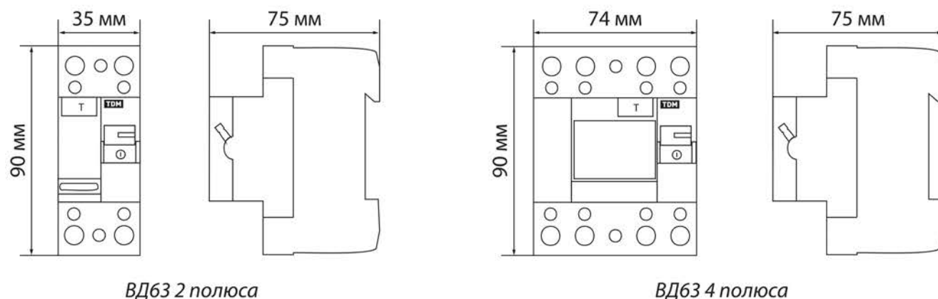
Рисунок 1. Габаритные размеры ВД63 2 полюса и ВД63 4 полюса
