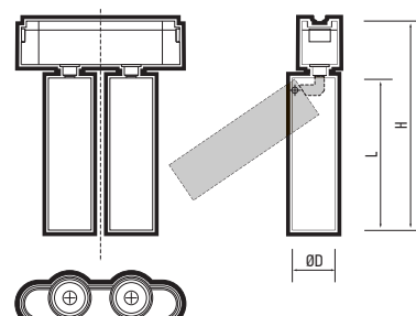
MTR16 2016 2x8w
