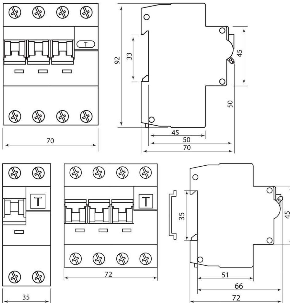
Рисунок 1. Габаритные размеры, мм
