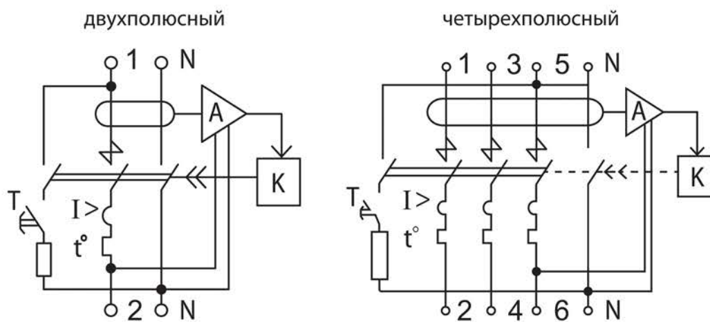
Рисунок 2. Схема подключения
