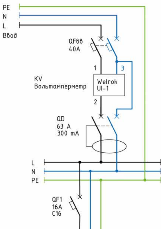
Схема 1. Вариант электрической схемы
