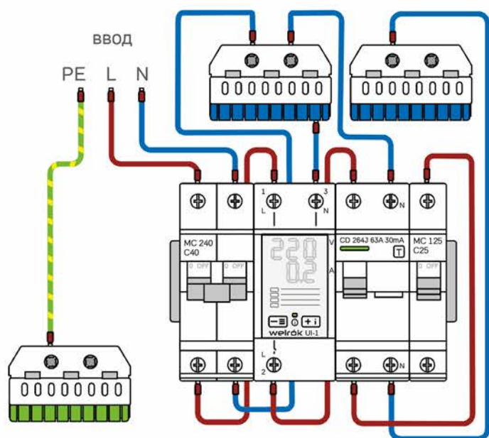
Схема 2. Вариант монтажной схемы
