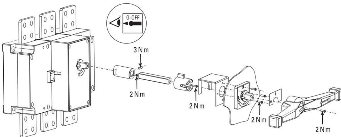
Рисунок 14а – Монтаж выносной ручки для рубильников 1000-1600 А
