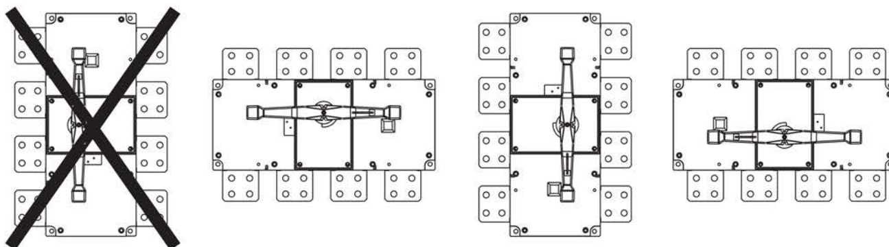
Рисунок 9б – Рабочее положение рубильников PowerSwitch 1000-2500 А
