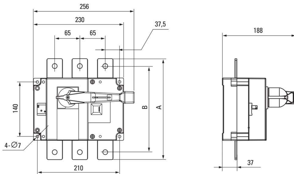
Рисунок 3а – Монтажные размеры рубильника PowerSwitch 400-630 А трехполюсного
