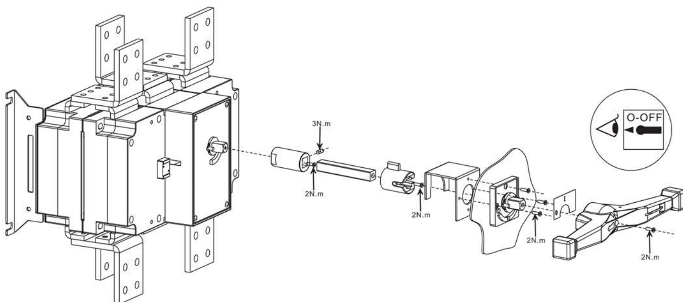
Рисунок 15а – Монтаж выносной ручки для рубильников 2000-3150 А
