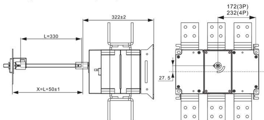
Наружные монтажные размеры
