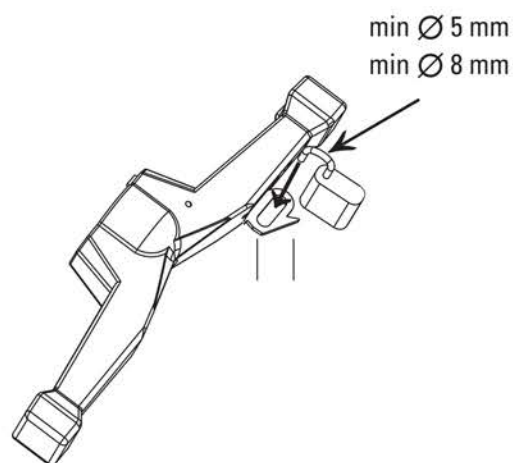
Рисунок 11б – Блокировка ручки рубильников 1000-1600 А навесным замком
