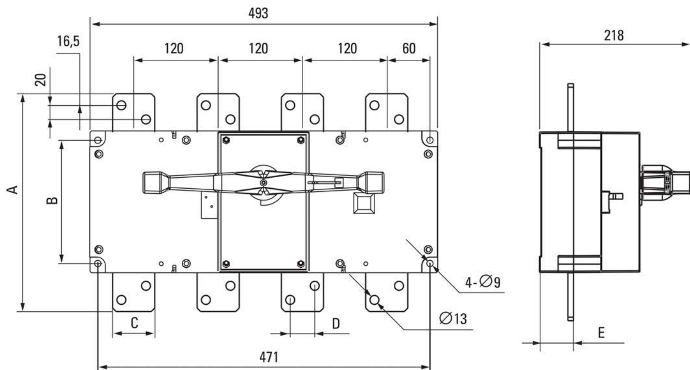
Рисунок 4б – Монтажные размеры рубильника PowerSwitch 1000-1600 А четырехполюсного
