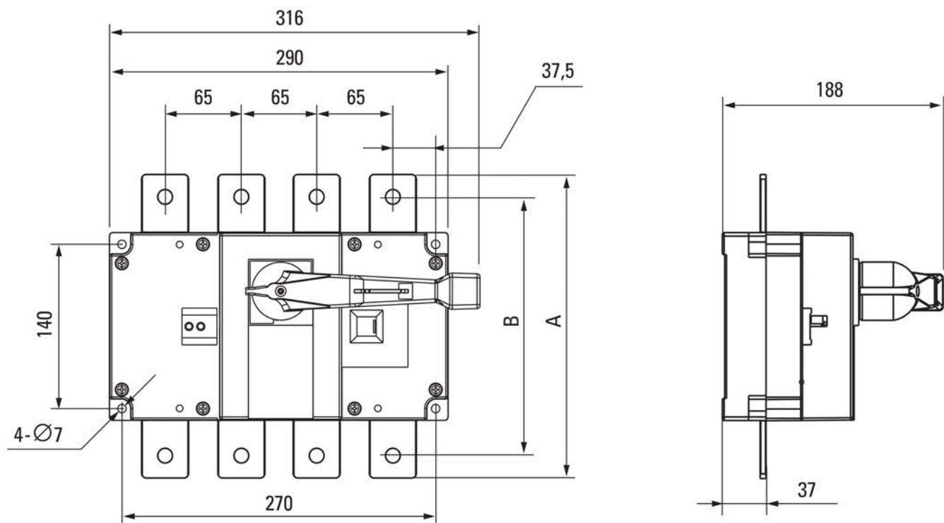
Рисунок 3б – Монтажные размеры рубильника PowerSwitch 400-630 А четырехполюсного
