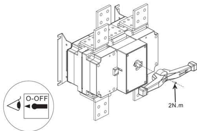
Рисунок 12а – Монтаж ручки на корпус рубильников 2000-3150 А
