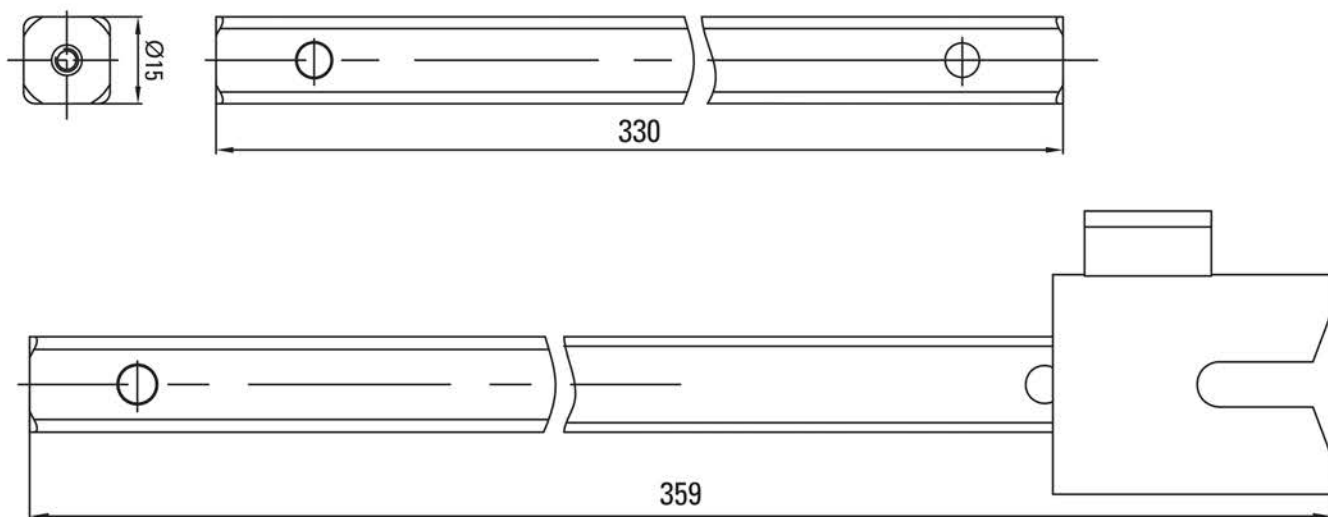
Рисунок 7б – габаритные чертежи штока ( 800~3150А)
