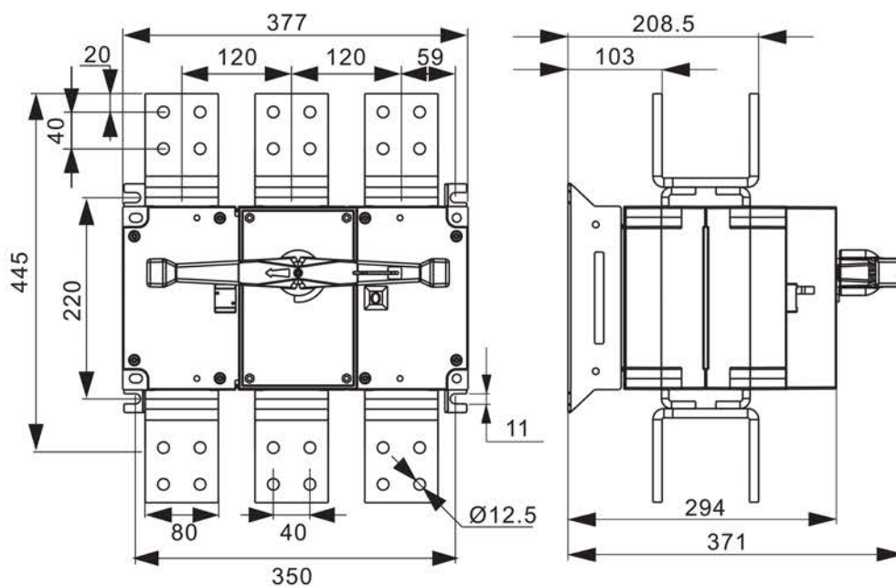
Рисунок 5а – Монтажные размеры рубильника PowerSwitch 2000-2500 А трехполюсного
