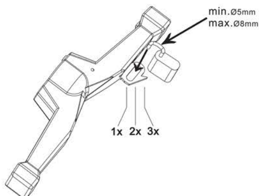
Рисунок 12б – Блокировка ручки рубильников 2000-3150 А навесным замком
