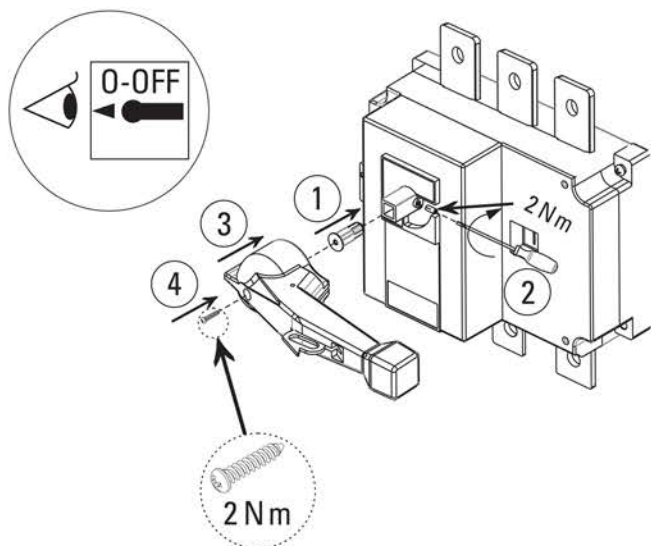
Рисунок 10а – Монтаж ручки на корпус рубильников 160-630 А
