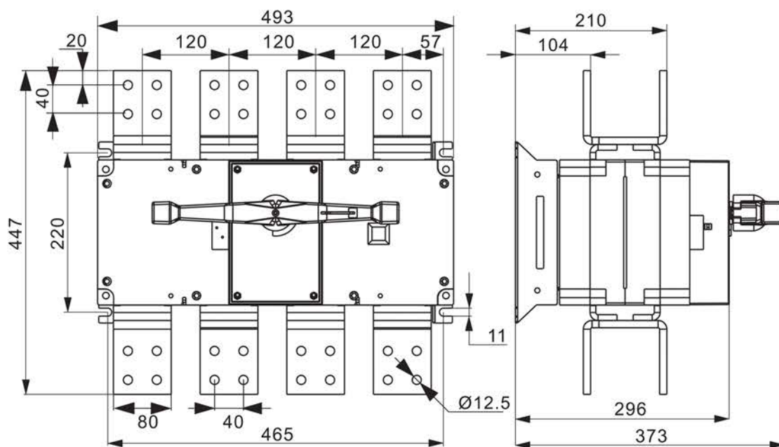
Рисунок 5б – Монтажные размеры рубильника PowerSwitch 2000-2500 А четырехполюсного
