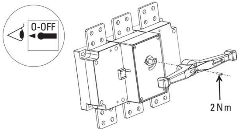
Рисунок 11а – Монтаж ручки на корпус рубильников 1000-1600 А
