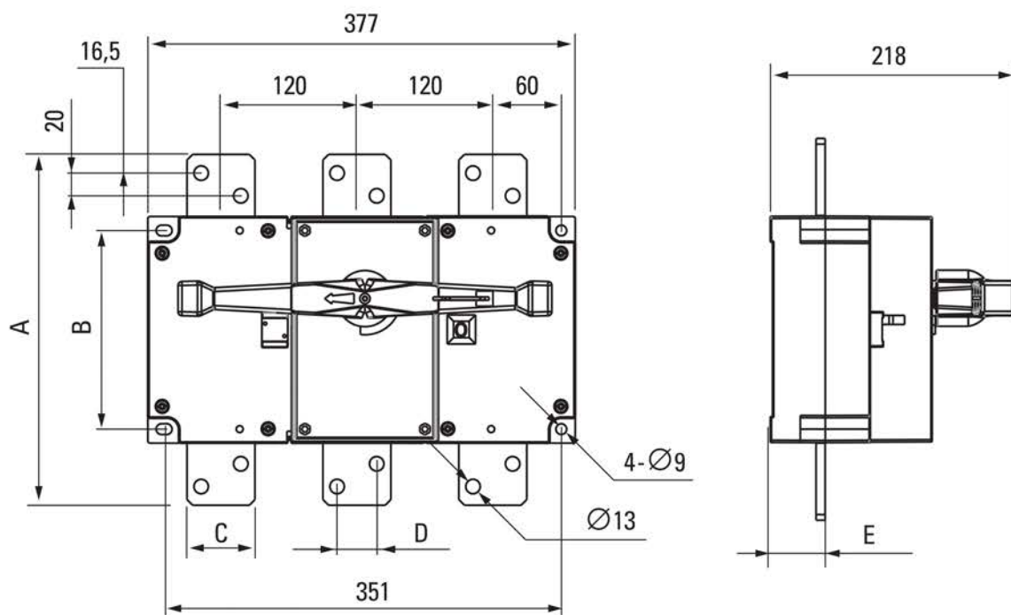
Рисунок 4а – Монтажные размеры рубильника PowerSwitch 1000-1600 А трехполюсного
