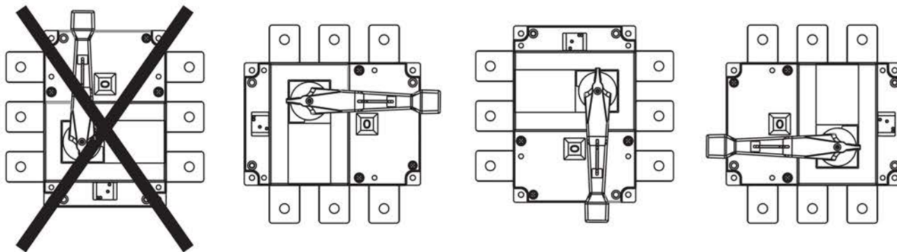
Рисунок 9а – Рабочее положение рубильников PowerSwitch 160-630 А
