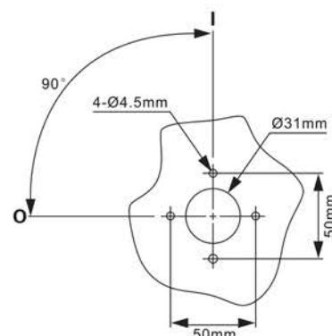
Монтажные размеры для двери шкафа
