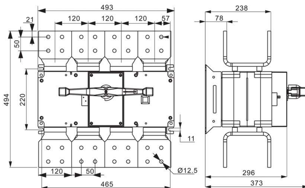
Рисунок 6б – Монтажные размеры рубильника PowerSwitch 3150 А четырёхполюсного
