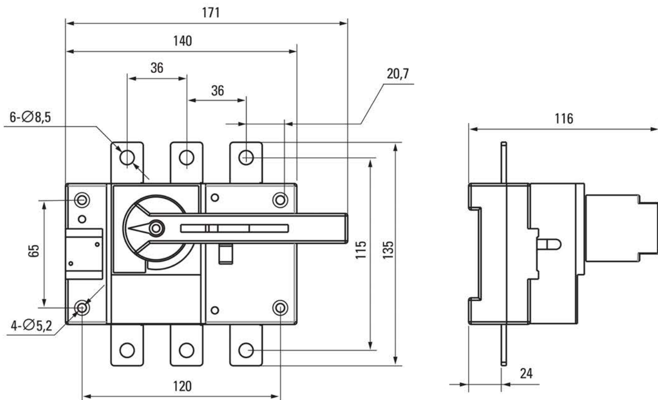
Рисунок 1а – Монтажные размеры рубильника PowerSwitch 160 А трехполюсного
