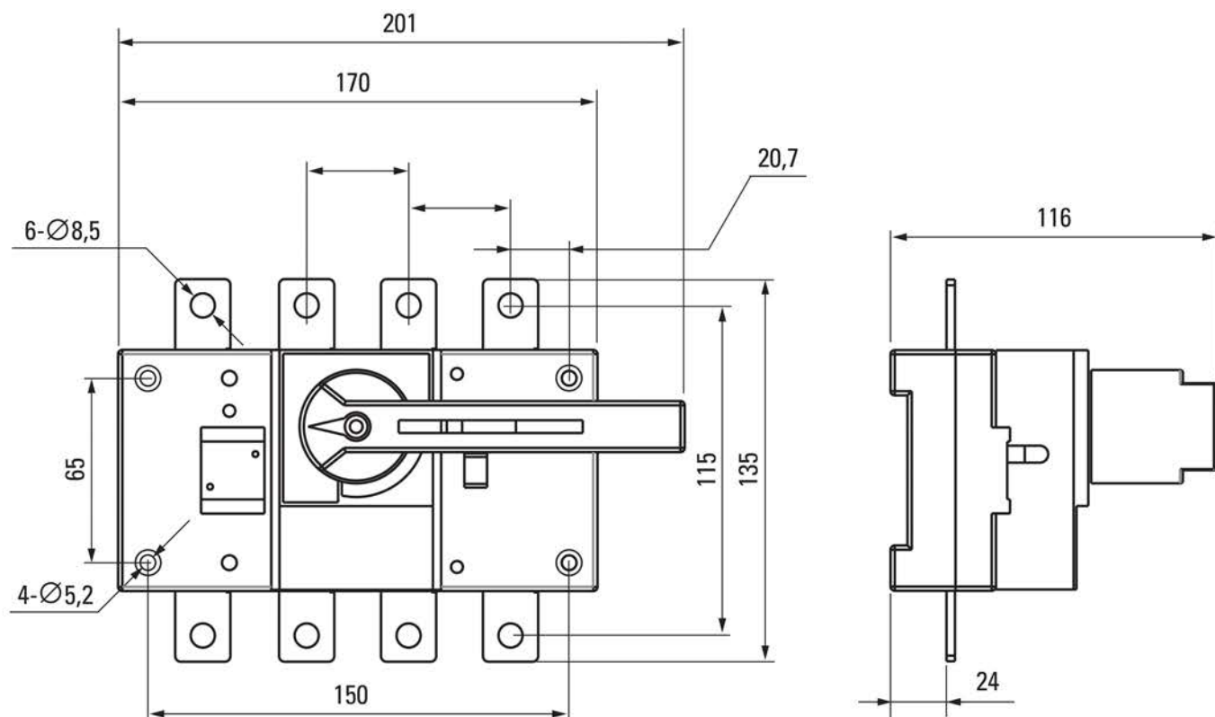
Рисунок 1б – Монтажные размеры рубильника PowerSwitch 160 А четырехполюсного
