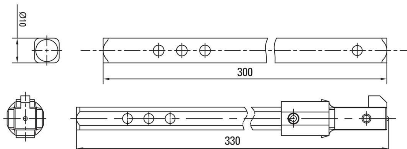
Рисунок 7а – габаритные чертежи штока (160~630А)
