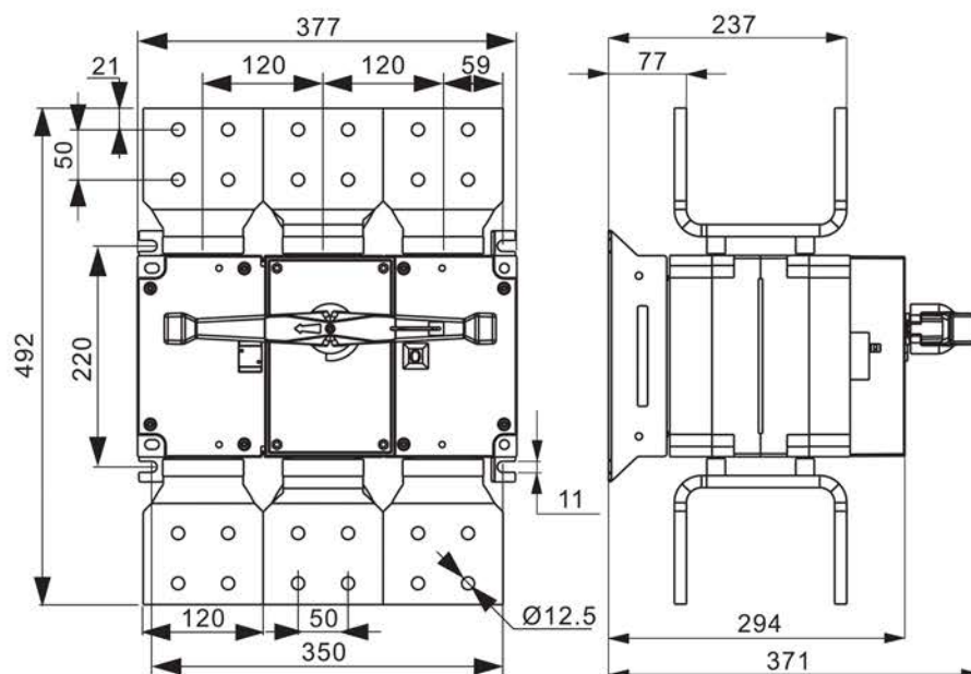
Рисунок 6а – Монтажные размеры рубильника PowerSwitch 3150 А трехполюсного
