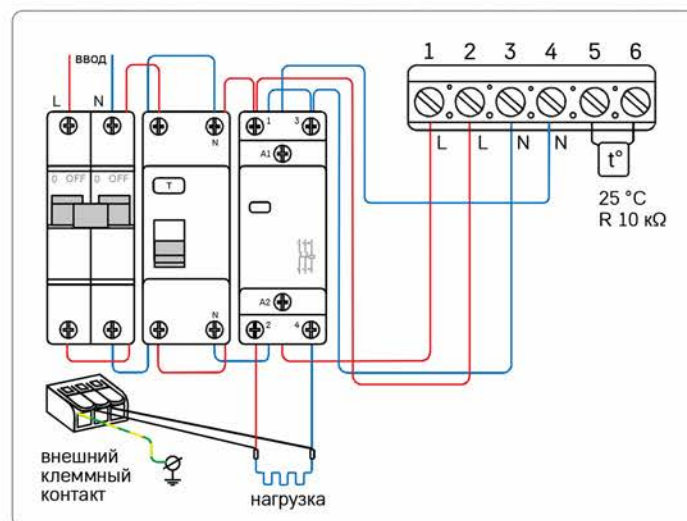
Схема 2. Схема подключения через магнитный пускатель
