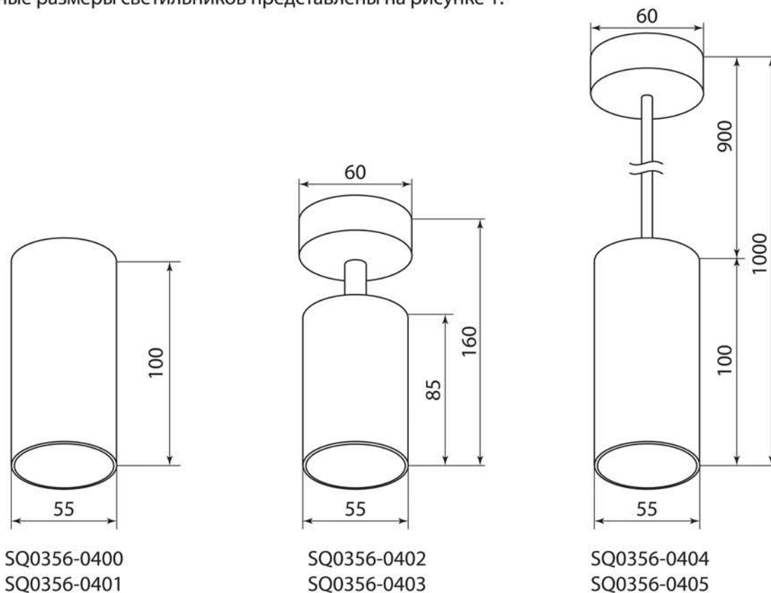
Рисунок 1. Габаритные размеры светильников, мм
