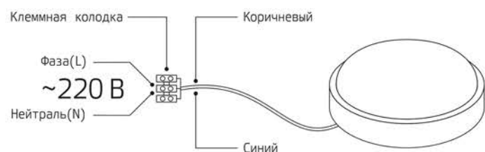
Рис. 1. Схема подключения светильника к электросети 220 В
