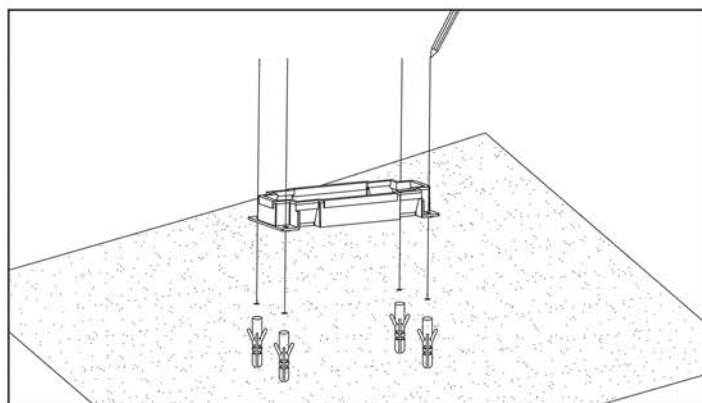
Рисунок 3. Подготовьте монтажные отверстия на поверхности грунта
