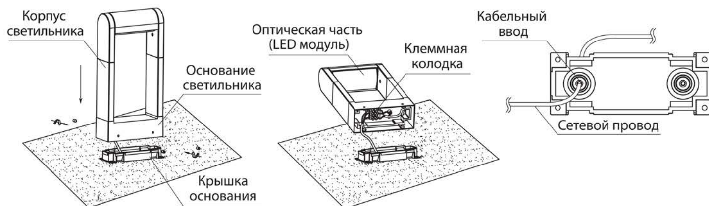
Рисунок 1. Конструкция светильника
