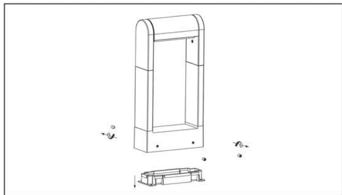
Рисунок 4. Отсоедините крышку основания светильника (открывается шестигранником)
