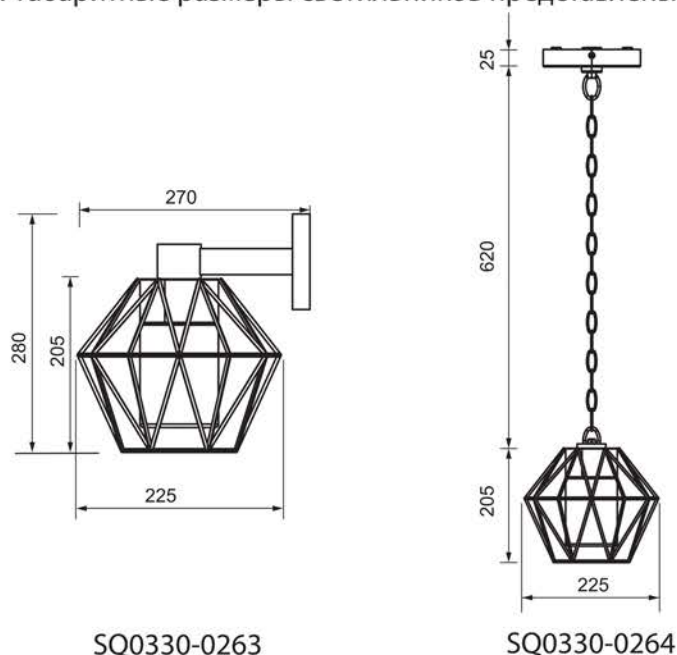
Рисунок 1. Габаритные размеры светильников, мм
