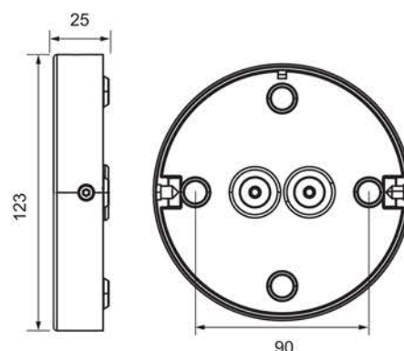
Рисунок 2. Основание светильника
