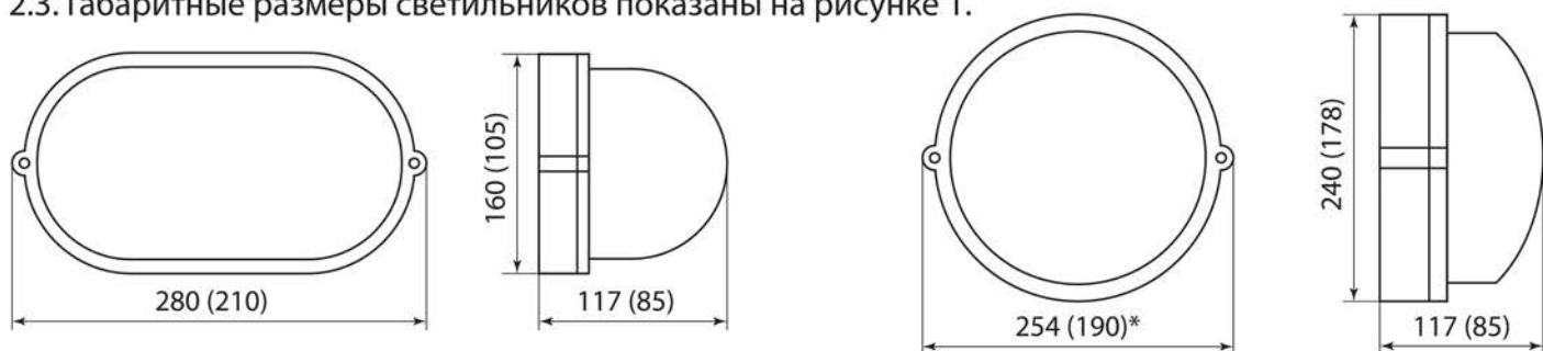
Рисунок 1. Габаритные размеры, мм
