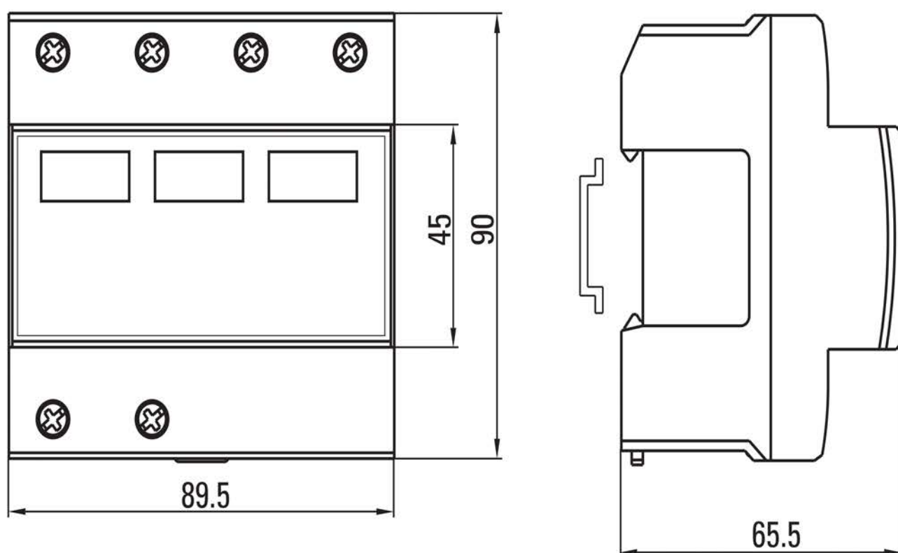
Рис. 7 - Габаритные и установочные размеры
