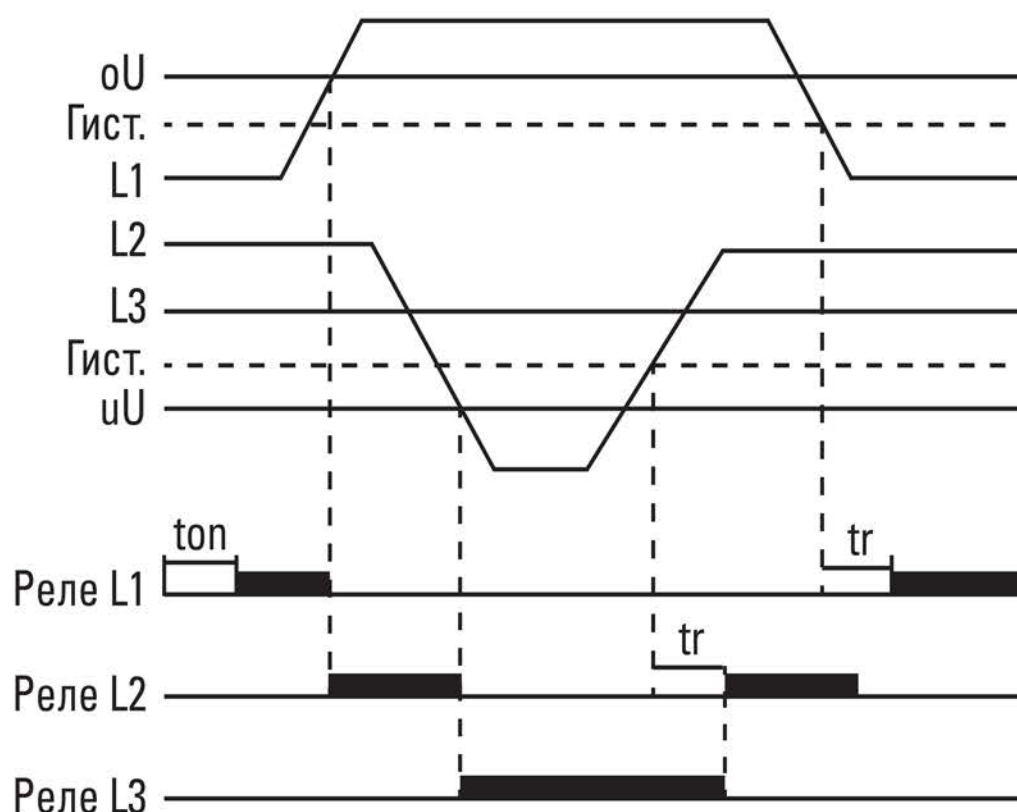
Рис. 1 - Диаграммы работы реле с задержкой возврата к приоритетной фазе (5-200с)
