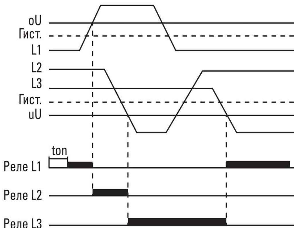
Рис. 2 - Диаграммы работы реле без возврата к приоритетной фазе
