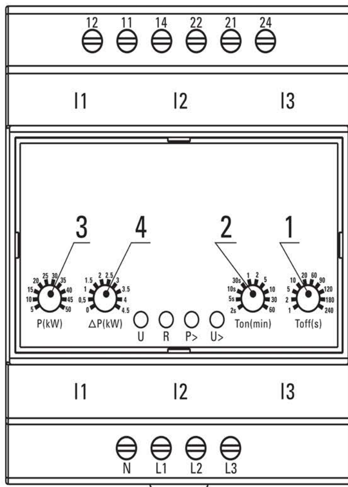
Рис. 3 — Органы управления и индикации
