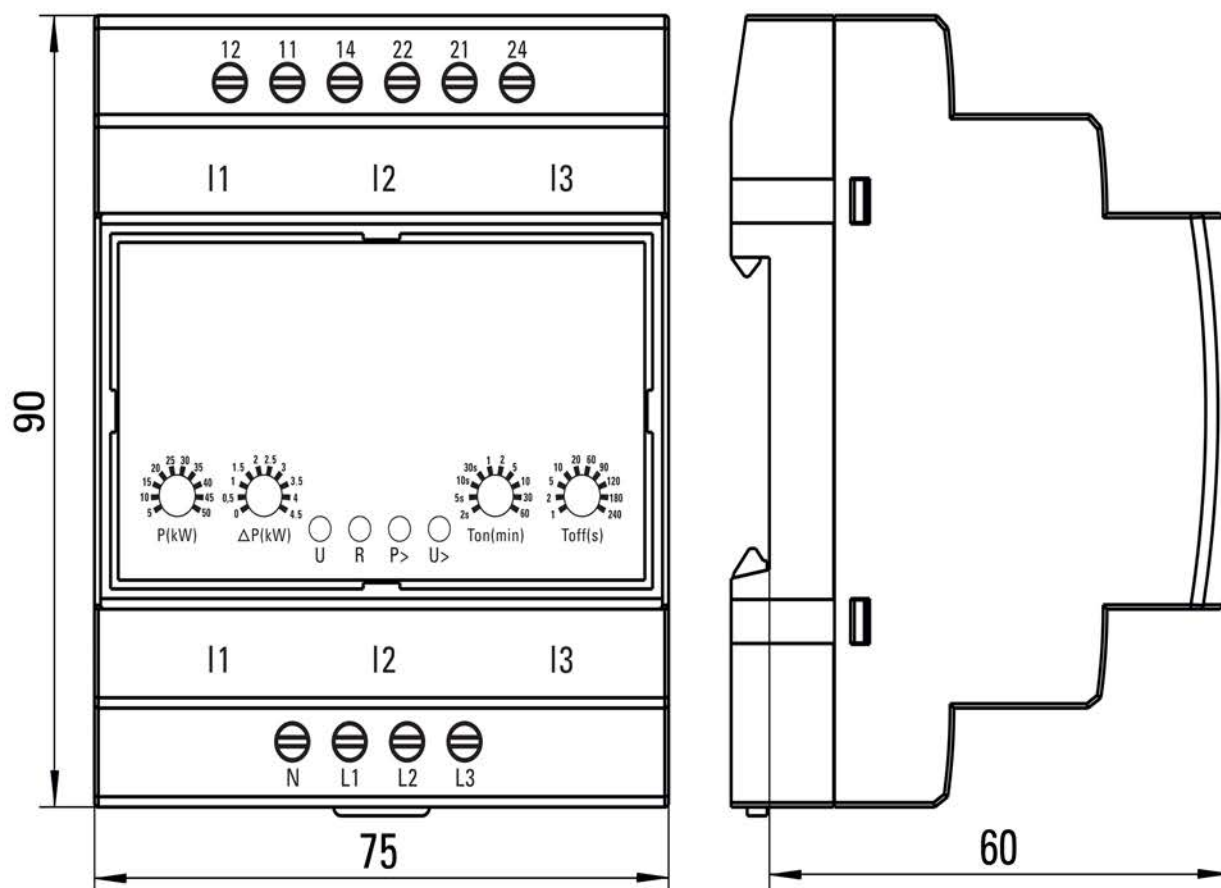
Рис. 4 — Габаритные и установочные размеры
