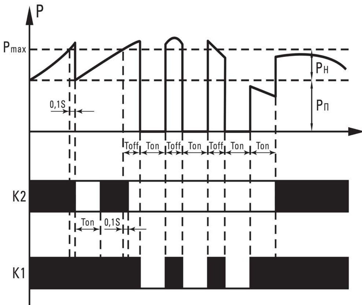
Рис. 1 — Диаграмма работы ограничителя с приоритетной нагрузкой
