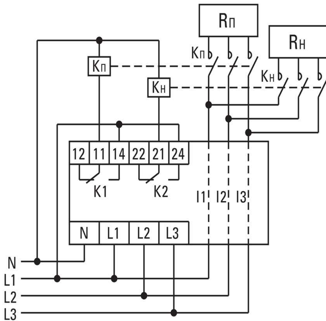
Рис. 2 — Схема подключения
