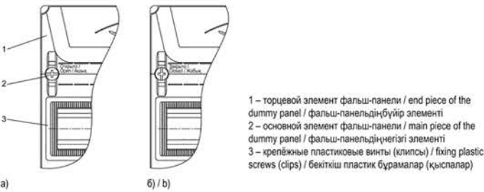
Рисунок / Figure / Сурет 1 – Оперативная панель / Faceplate / Жедел панель
