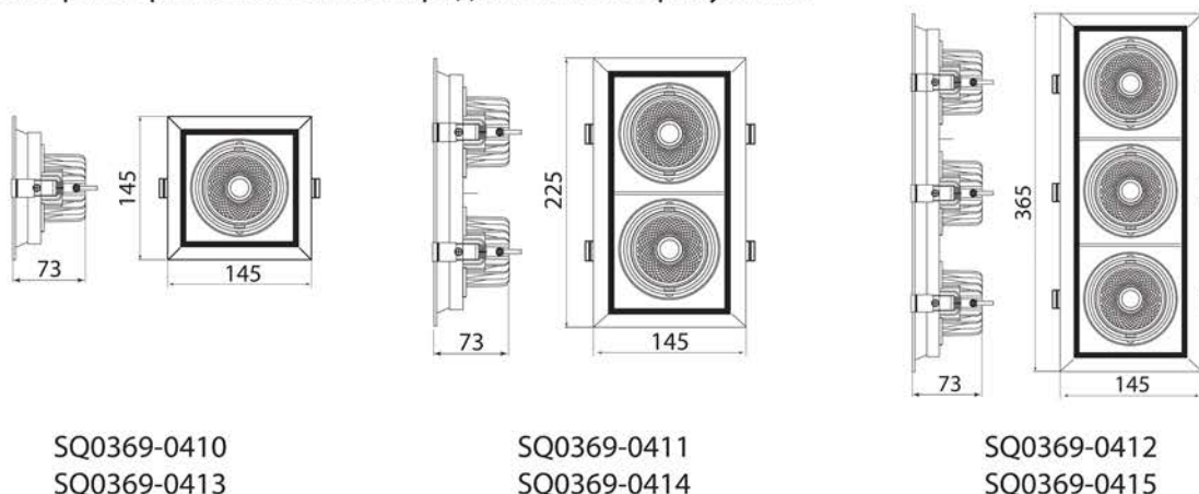
Рисунок 1. Габаритные размеры светильников, мм
