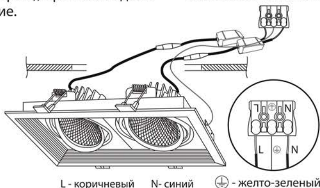
Рисунок 2. Подключение светильника с драйвером к электрической сети
