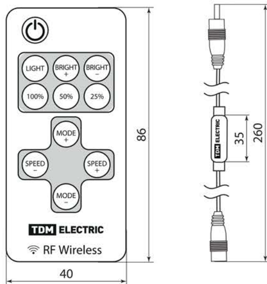
Рисунок 1. Габаритные размеры диммера, мм
