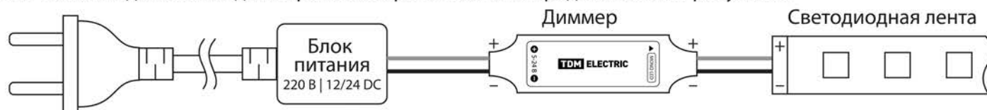
Рисунок 2. Схема подключения диммера
