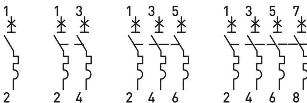
Рис. 3. Схемы подключения
