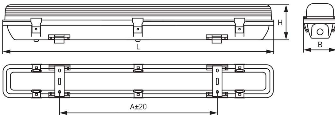
Рис. 1 - Габаритные размеры
