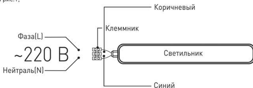
Рис.1. Схема подключения светильника к сети 220В.
