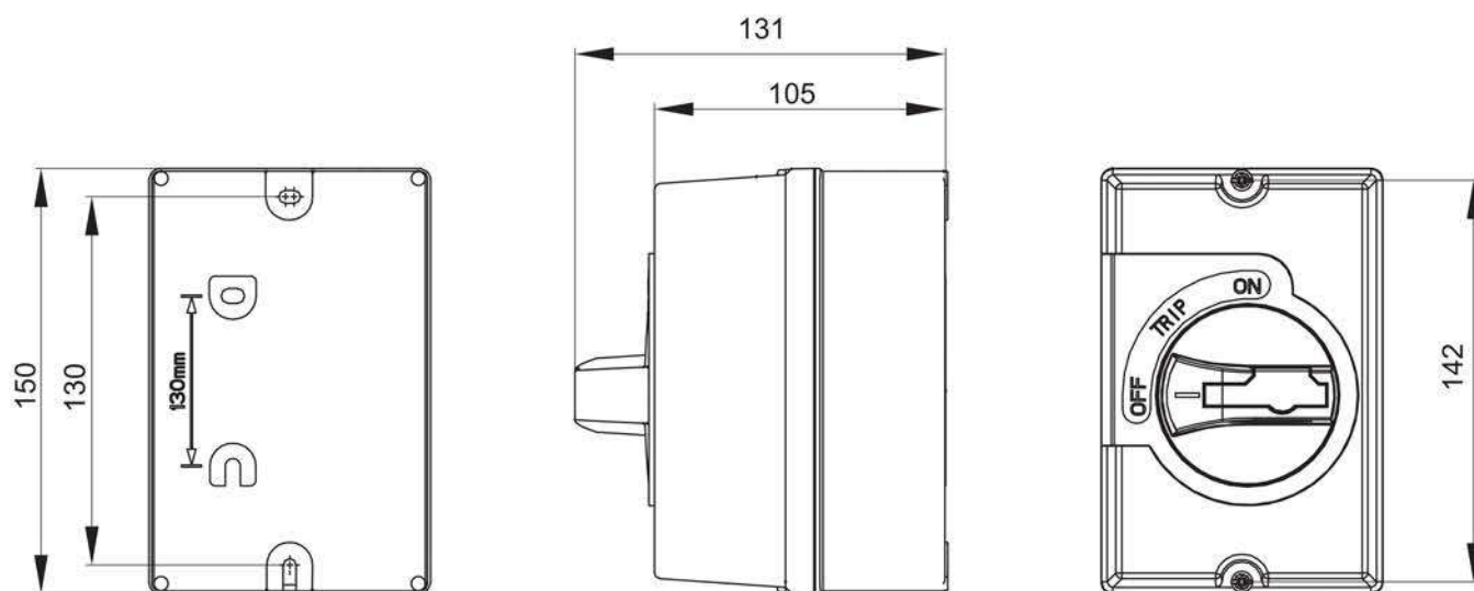
Рисунок 7 – Габаритные и установочные размеры оболочки
