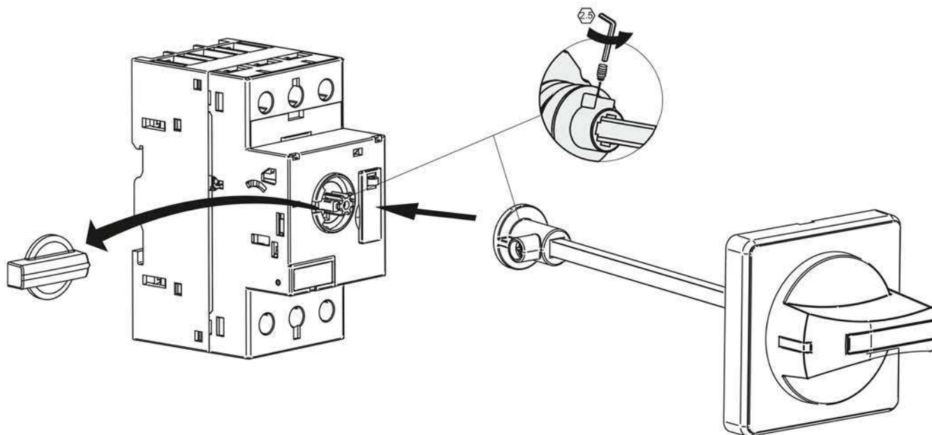
Рисунок 13 – Монтаж поворотной рукоятки на выключатель
