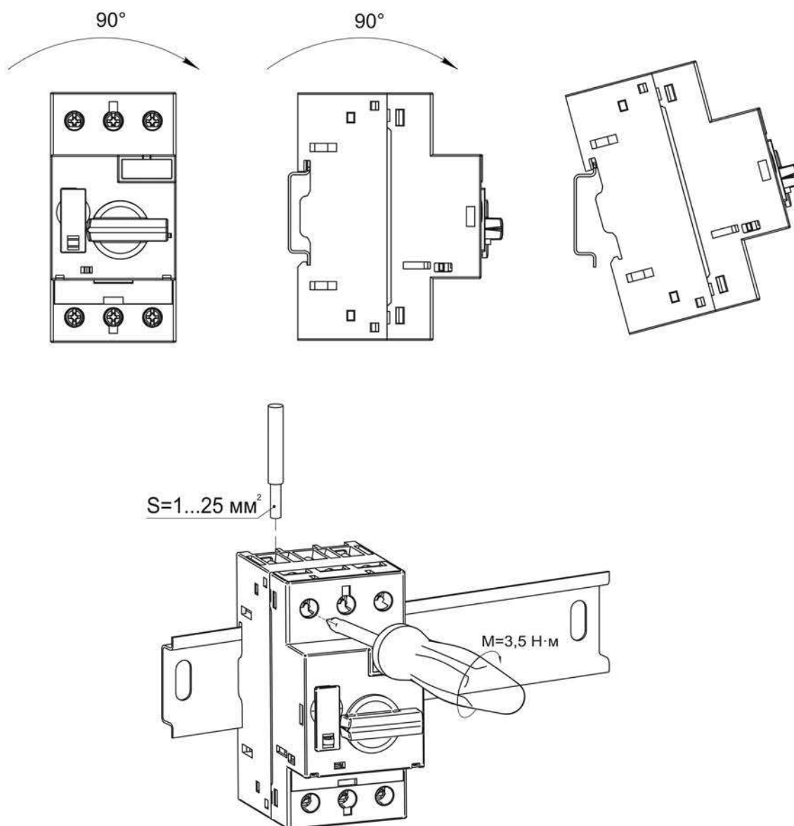
Рисунок 9 – Монтаж выключателя
