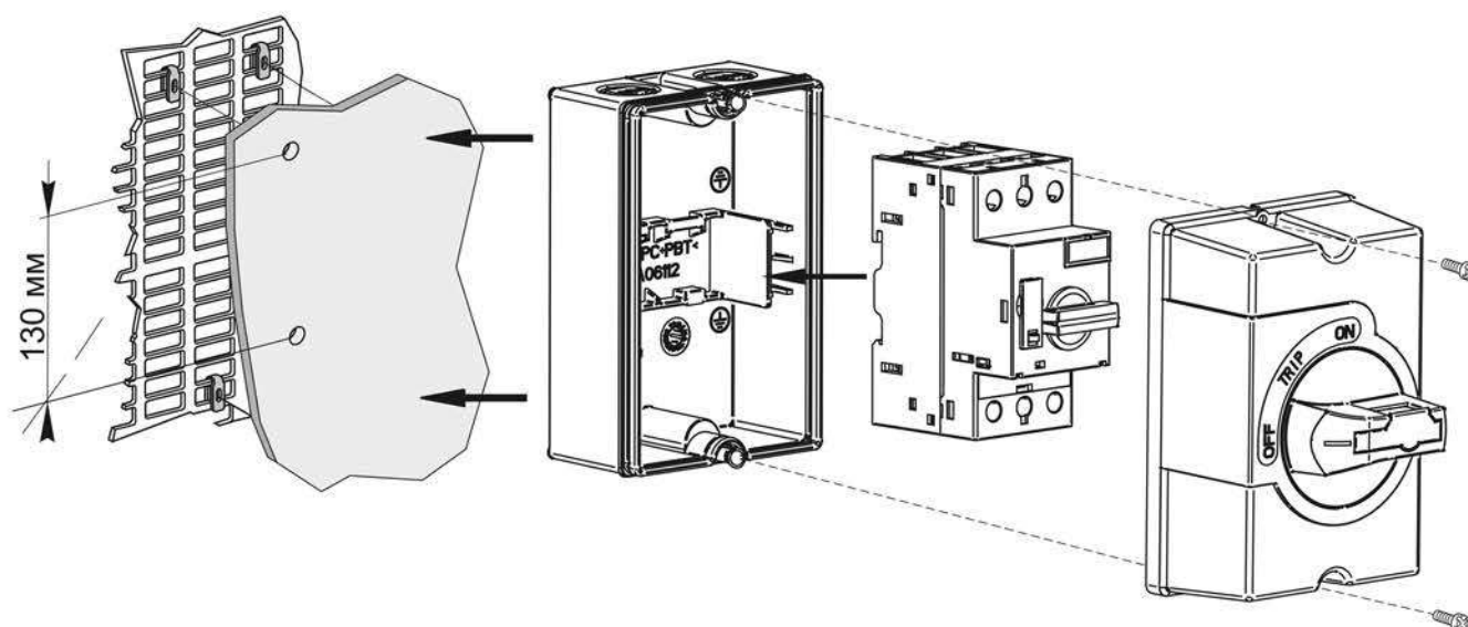
Рисунок 12 – Монтаж оболочки и установка выключателя
