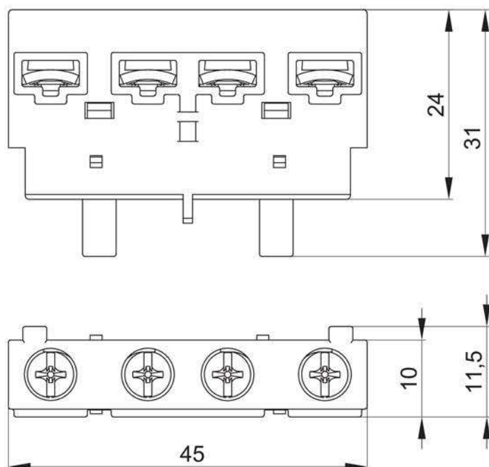
Рисунок 5 – Габаритные и установочные размеры контактов поперечных
