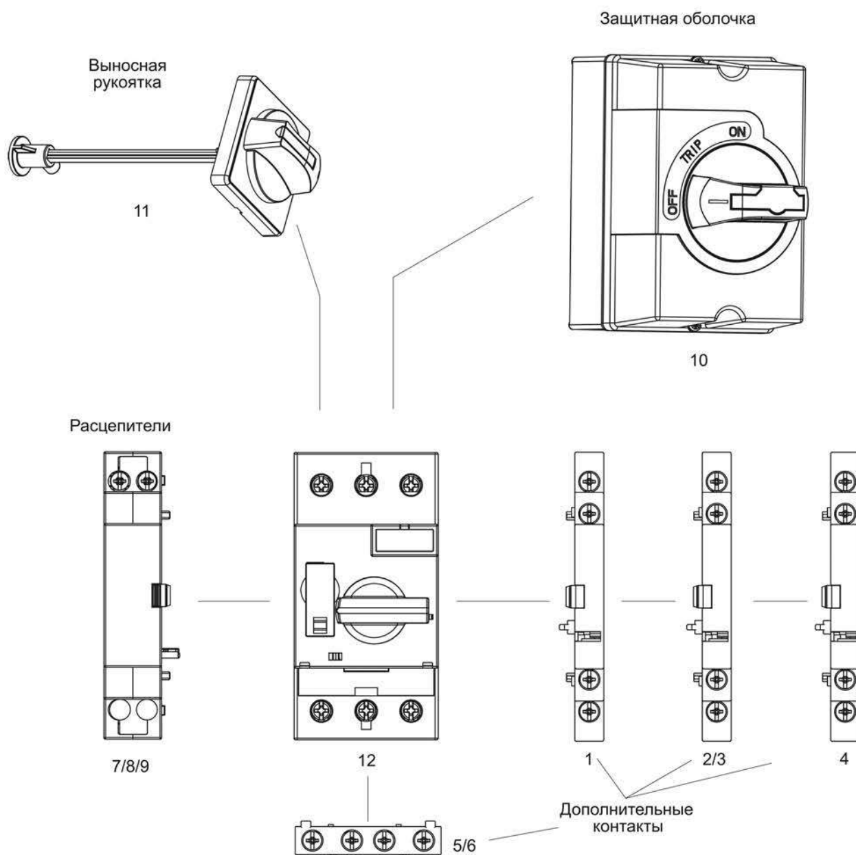
Рисунок 8 – Разнесенная сборка
