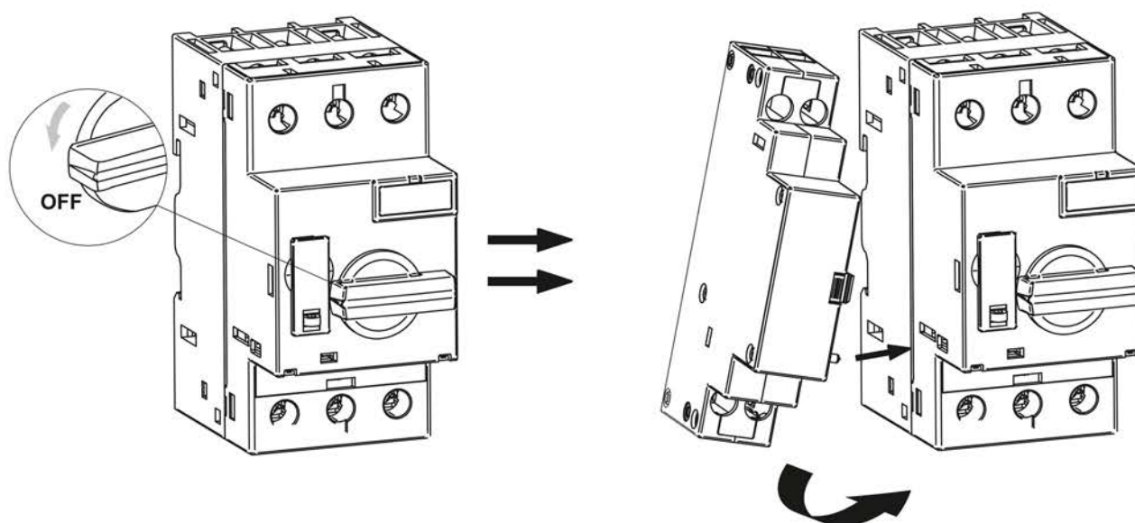
Рисунок 10 – Монтаж расцепителей
