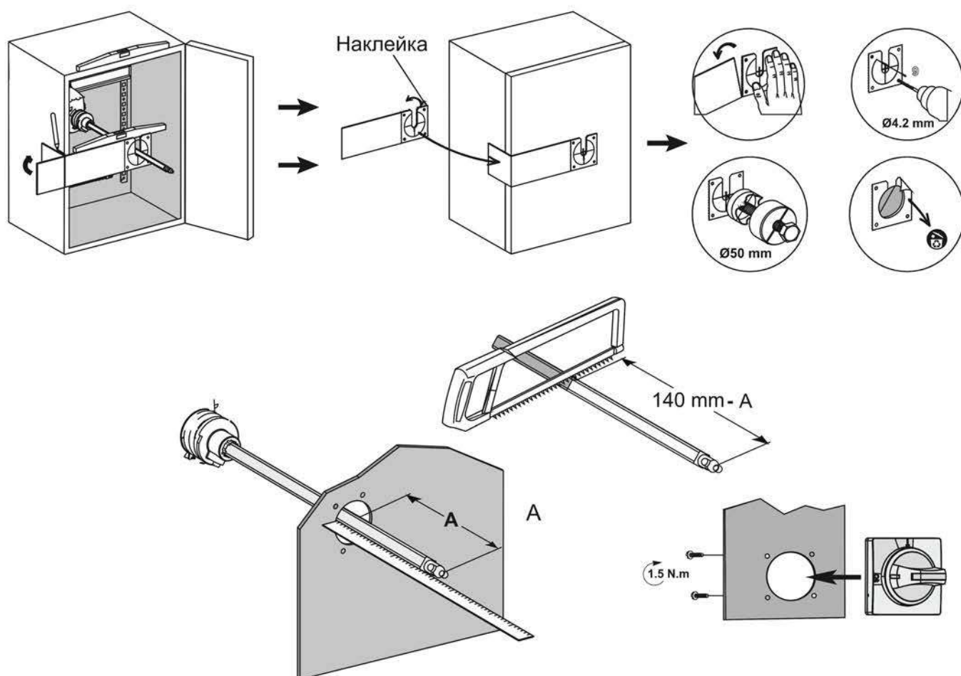
Рисунок 14 – Монтаж поворотной рукоятки на дверцу распределительного шкафа
