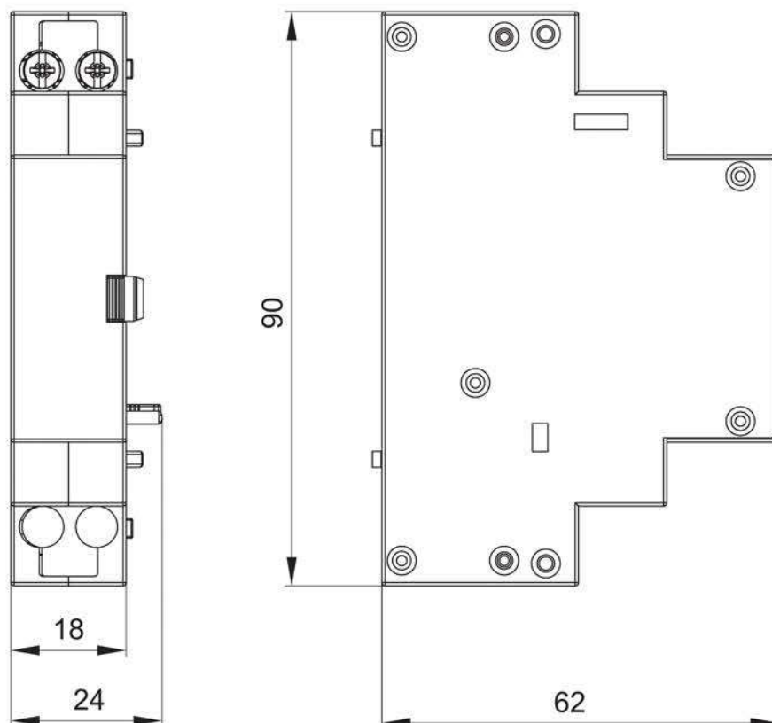
Рисунок 3 – Габаритные и установочные размеры расцепителей
