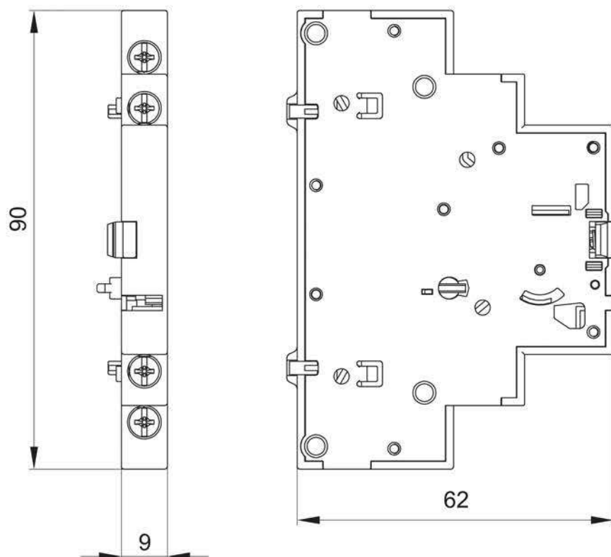
Рисунок 4 – Габаритные и установочные размеры контактов боковых
