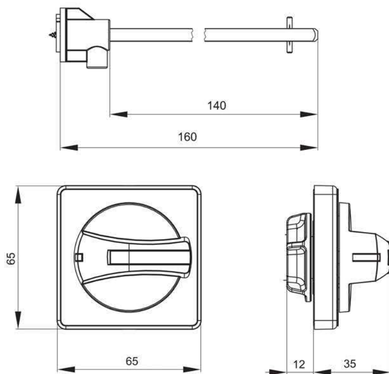
Рисунок 6 – Габаритные и установочные размеры поворотной рукоятки
