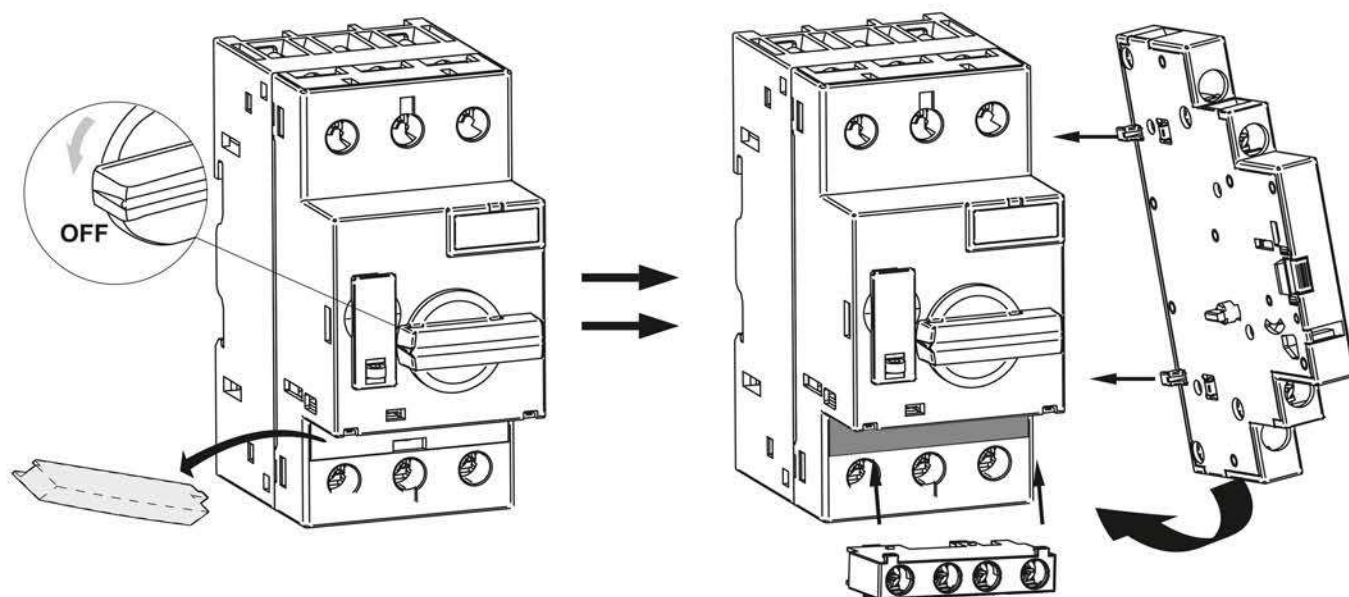
Рисунок 11 – Монтаж контактов
