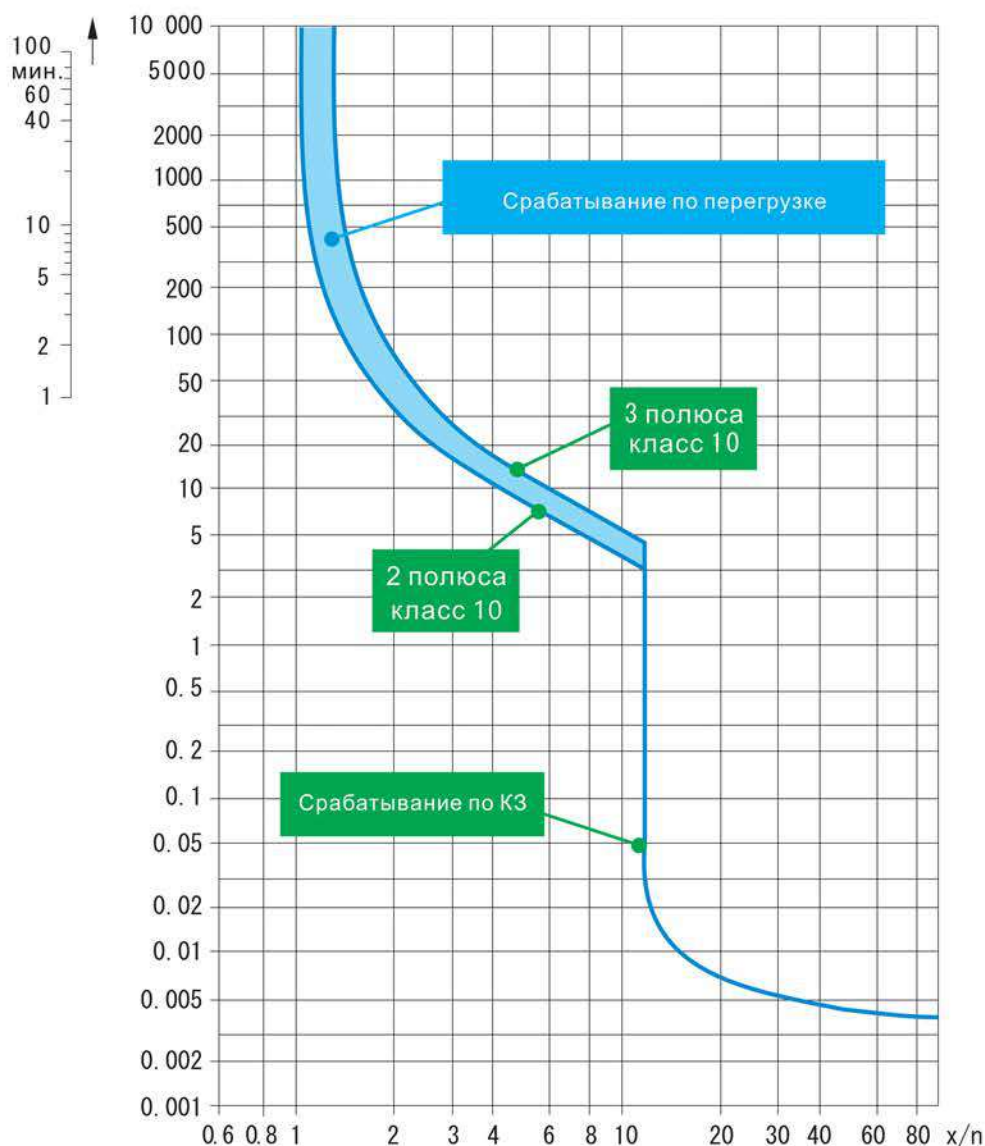
Рисунок 2 – Время – токовые характеристики выключателей
