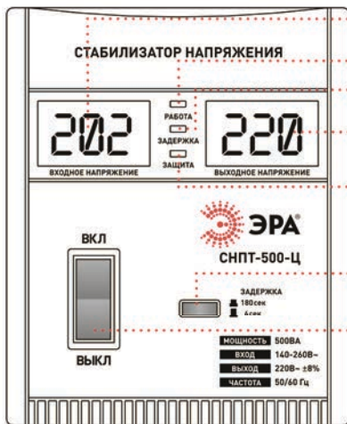
Модели СНПТ-500...2000-Ц
