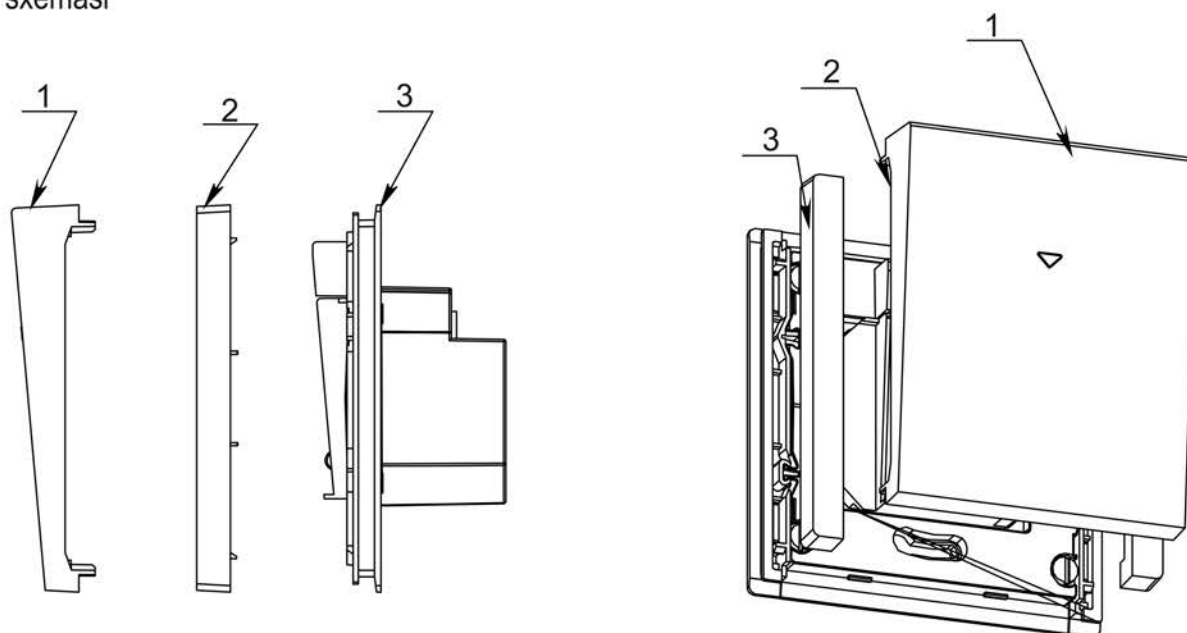
Рисунок 3 – Порядок монтажа выключателя / Figure 3 – Switch installation procedure / 3 сурет – Ажыратқышты монтаждау тәртібі / Figura 3 – Procedura de instalare a întrerupătorului / Зураг 3 - Унтраалгын суурилуулах дараалал / 3-rasm - Viklyuchatelni montaj qilish tartibi
