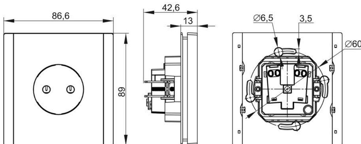
а) Розетка без контактов заземления / Socket without grounding contacts / Жерге түйықтау түйіспелері жоқ розеткалар / Prize fără contacte de împământare / Газардуулалт контактгүй залгуурууд / Yerga ulanish kontaktlariga ega bo'lmagan rozetkalar
