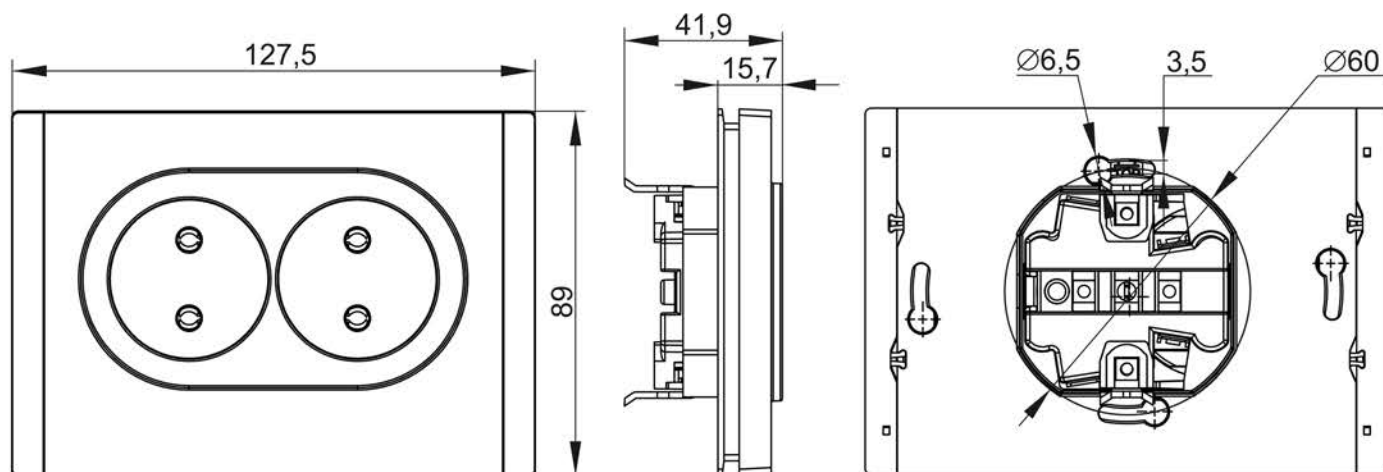
h) Розетка двухместная без контактов заземления / Double socket without grounding contacts / Жерге түйіспелерінсіз екі орынды розетка / Priză dublă fără contacte de împământare / Газардуулалт контактгүй давхар залгуурууд / Yerga ulanish kontaktlari mavjud bo'lmagan ikki o'rinli rozetka
