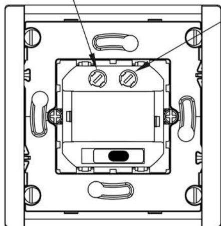
Рисунок 3 – Конструкция датчика движения / Figure 3 – Motion sensor design / 3 сурет – Қимыл датчигінің құрылымы / Figura 3 - Designul senzorului de mișcare / Зураг 3 - Хөдлөх бүртгэгчийн бүтээц / 3-rasm - Harakat sensorining konstruktsiyasi
