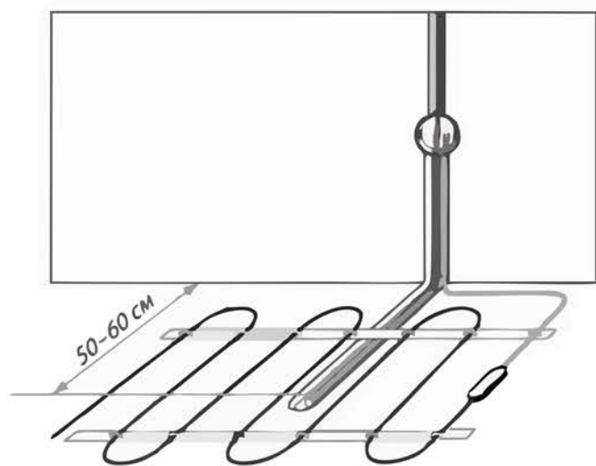
Рисунок 3- Монтаж терморегулятора / Figure 3 - Installation of the thermostat / 3 сурет – Термореттегішті монтаждау / Figura 3- Instalarea termostatlui / Зурар 3 - Терморегуляторын суурилуулах / 3-rasm - Termoregulyatorni montaj qilish
