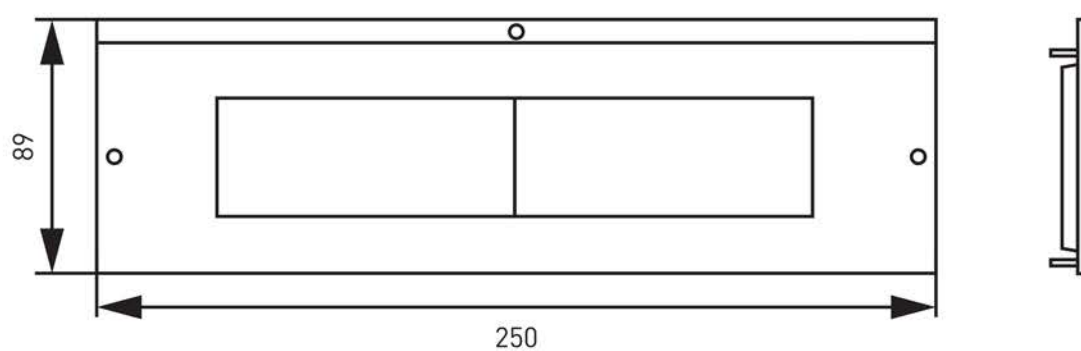
Рис. 9 – Рамка приборная сплошная (арт. cl-гр-0-24) / Рамка приборная классик на 3 места (арт. cl-гр-3-24) / Рамка приборная на 8 модулей (арт. cl-гр-4-24)
