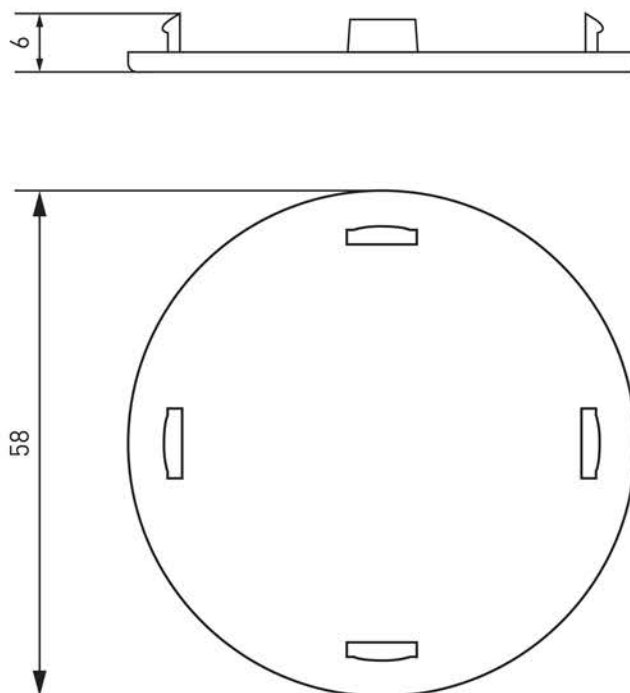
Рис. 11 – Заглушка круглая (арт. cl-z-0-24)
