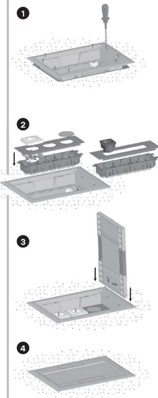
Рис. 17 – Установка лючка
