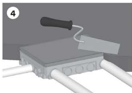
Рис. 16 – Порядок монтажа коробки напольной для лючка в бетонный пол
