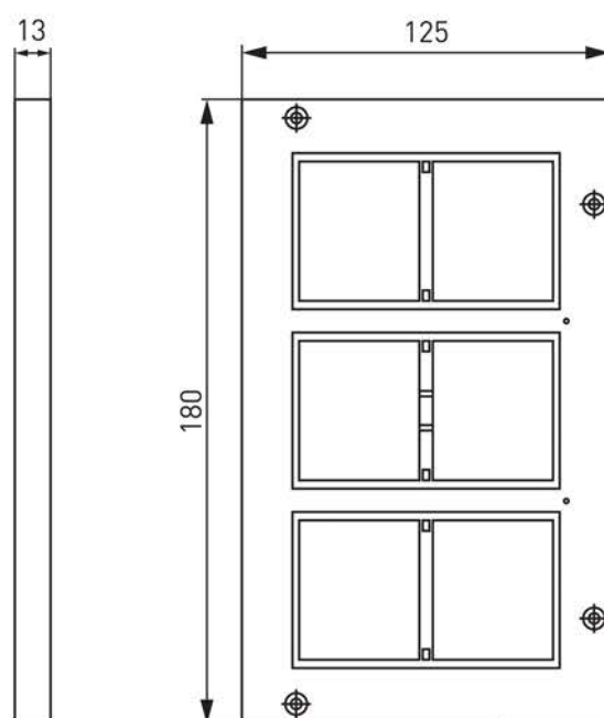
Рис. 12 – Рамка приборная на 12 модулей (арт. cl-рр-12-24)
