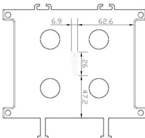
Рис. 14 – Лючок напольный IP66 C-Line WP-6 (арт. cl-lnwp-6)
