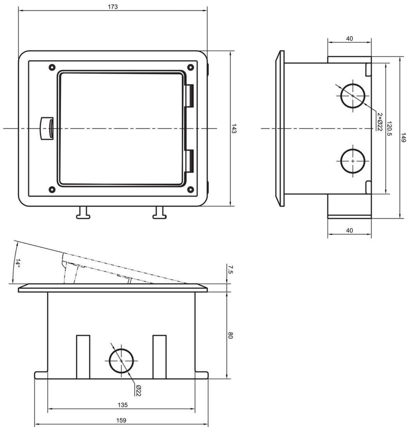
Рис. 14 – Лючок напольный IP66 C-Line WP-6 (арт. cl-lnwp-6)
