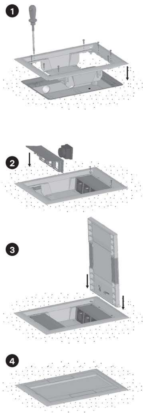
Рис. 17 – Установка лючка
