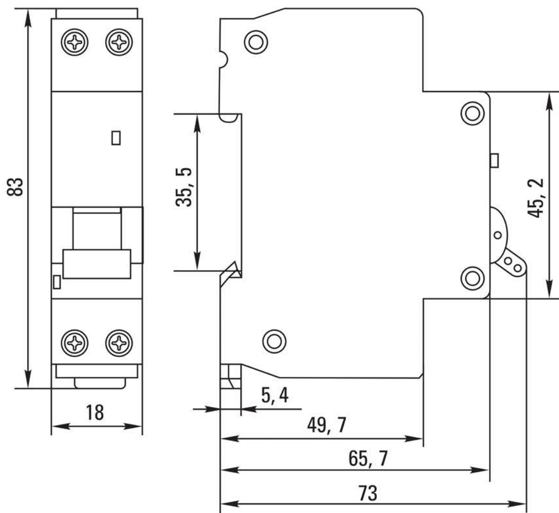
Рис. 4 – Габаритные размеры АВДТ-63
